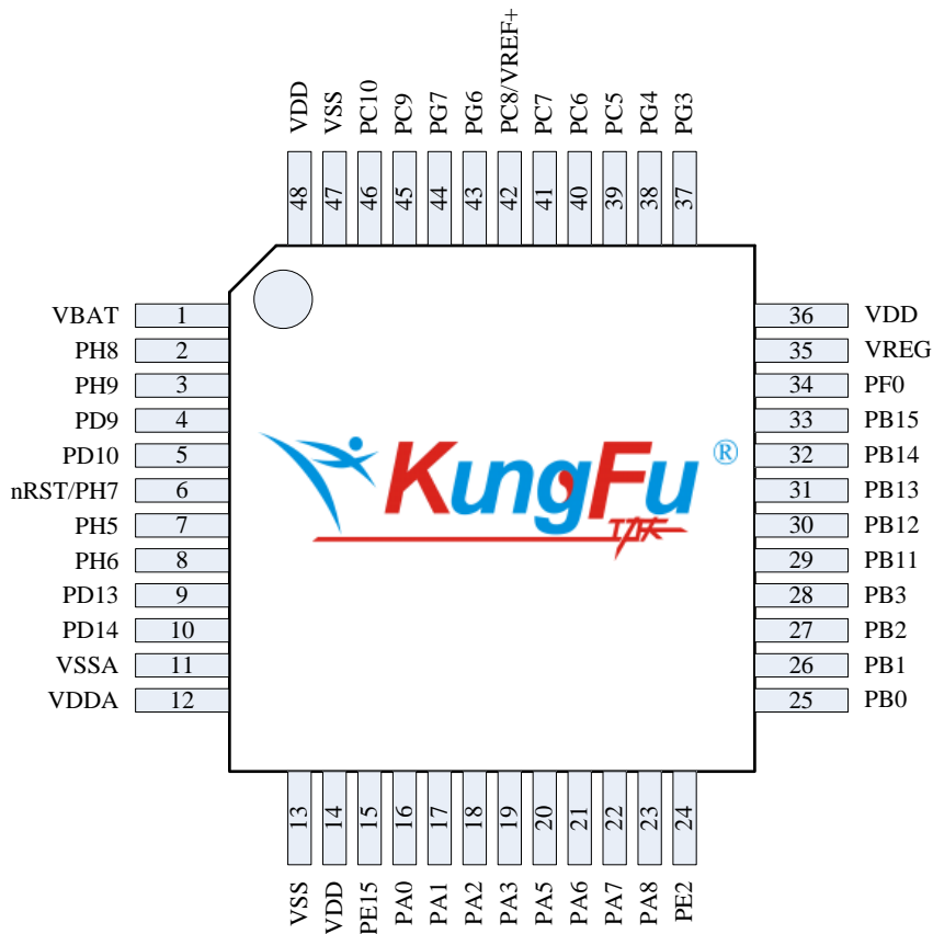
图 2-4 LQFP48
