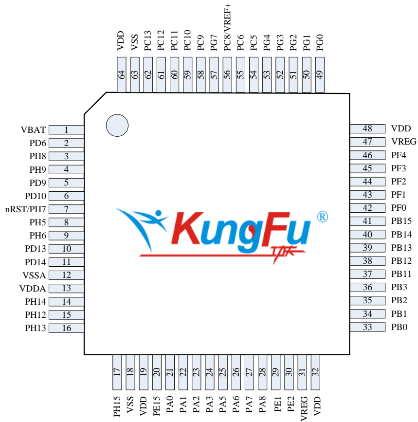
图 2-5 LQFP64
