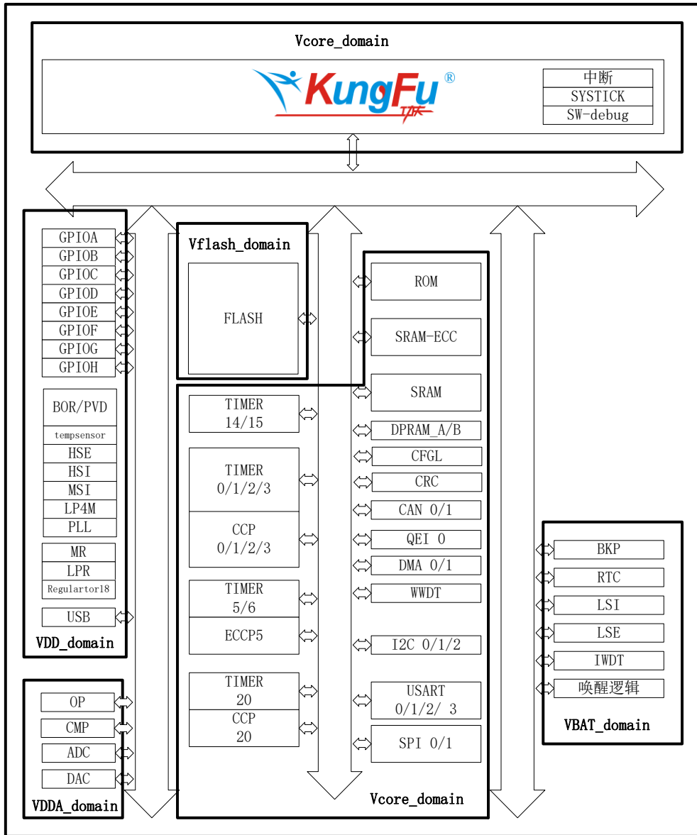
图 2-3 系统结构框图
