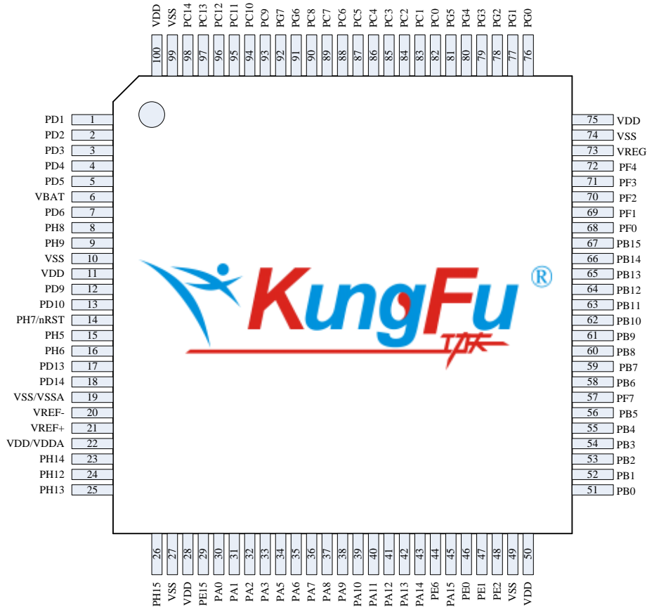
图 2-6 LQFP100
