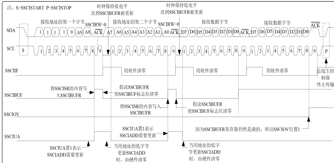
图 10.3 从动模式时序（接收，10 位地址）
