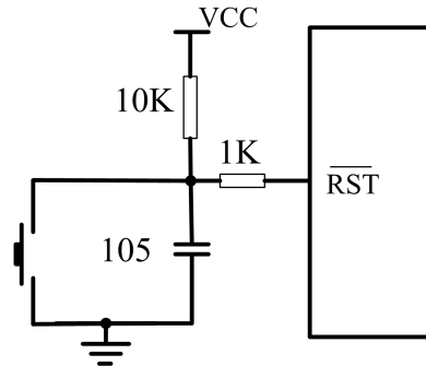
图 14.2 建议 \overline{\text{RST}} 复位电路
