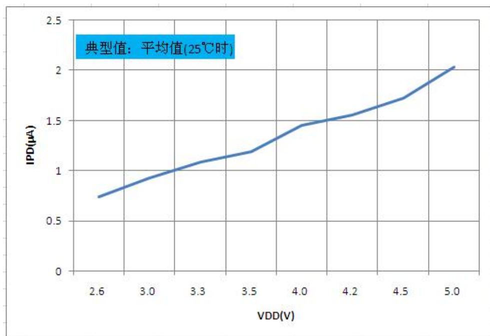
图18.2: 不同VDD 时典型IPD — VDD 关系曲线图
