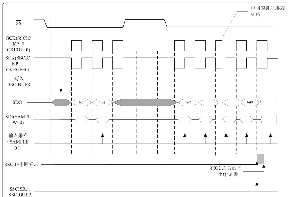
图10.31 从动时序图
