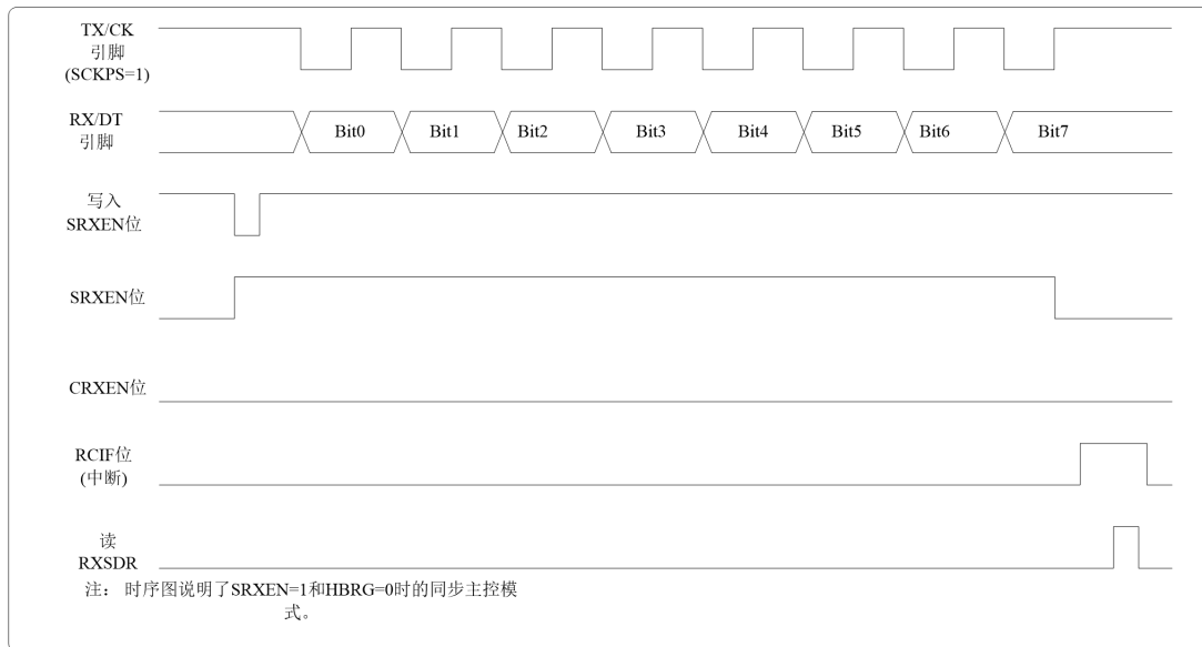
图 13.16 半双工同步接收（主控模式，SRXEN=1，SCKPS=1）
