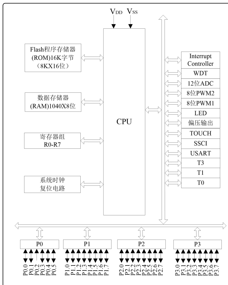
图 1.1 KF8TS2716 系统框图
