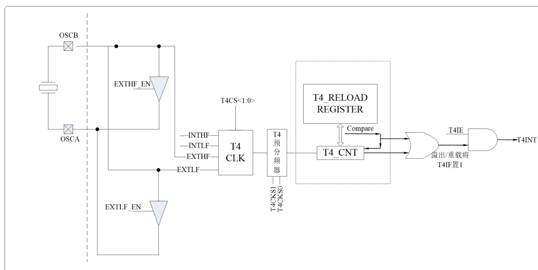
图 6.5 T4 原理框图
