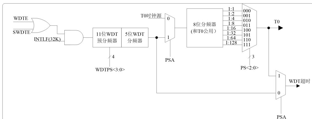
图 16.1 看门狗定时器框图
