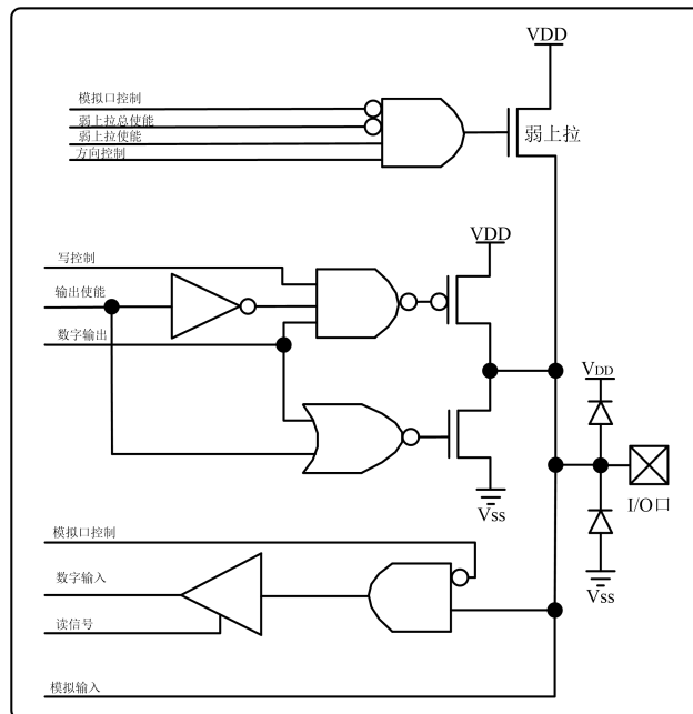
图 2.5 P2 口引脚原理功能框
