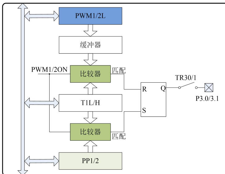
图 8.1 PWM1/2 逻辑框图
