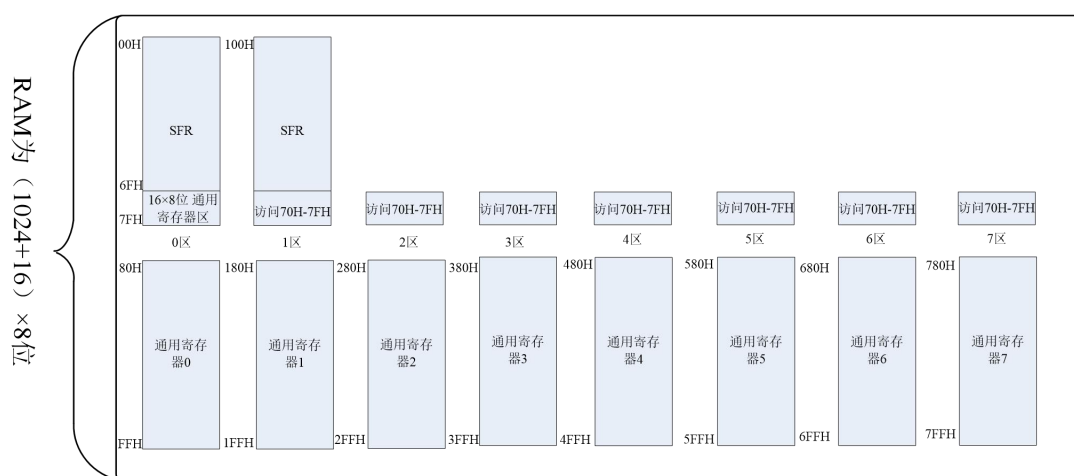
图 3.5 数据存储器地址映射图
