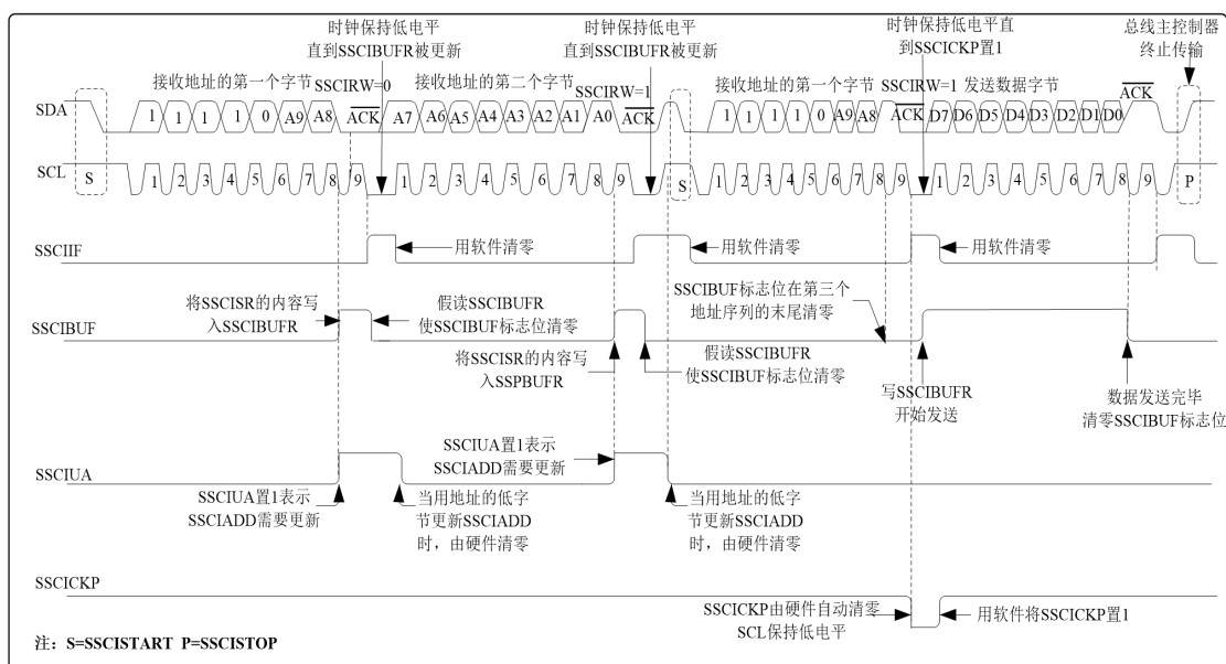
图 10.5 从动模式时序（发送，10 位地址）
