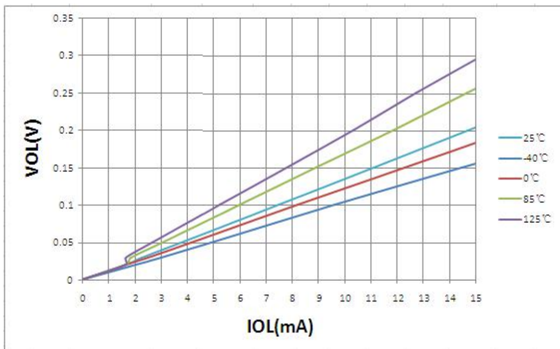
图18.9:不同温度时VOL — IOL 关系曲线图 (VDD = 5.0V)
