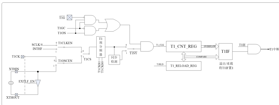
图 6.2 T1 原理框图
