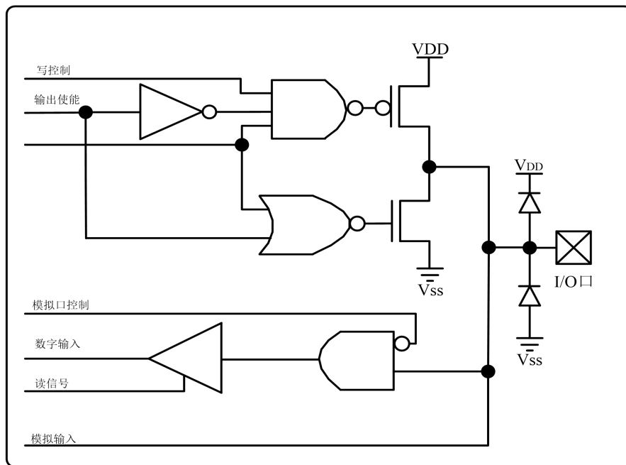
图 2.6 P3 口引脚原理功能框图
