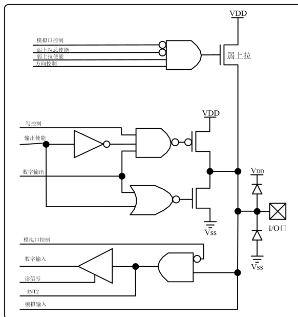
图 2.4 P1 口引脚原理功能框图
