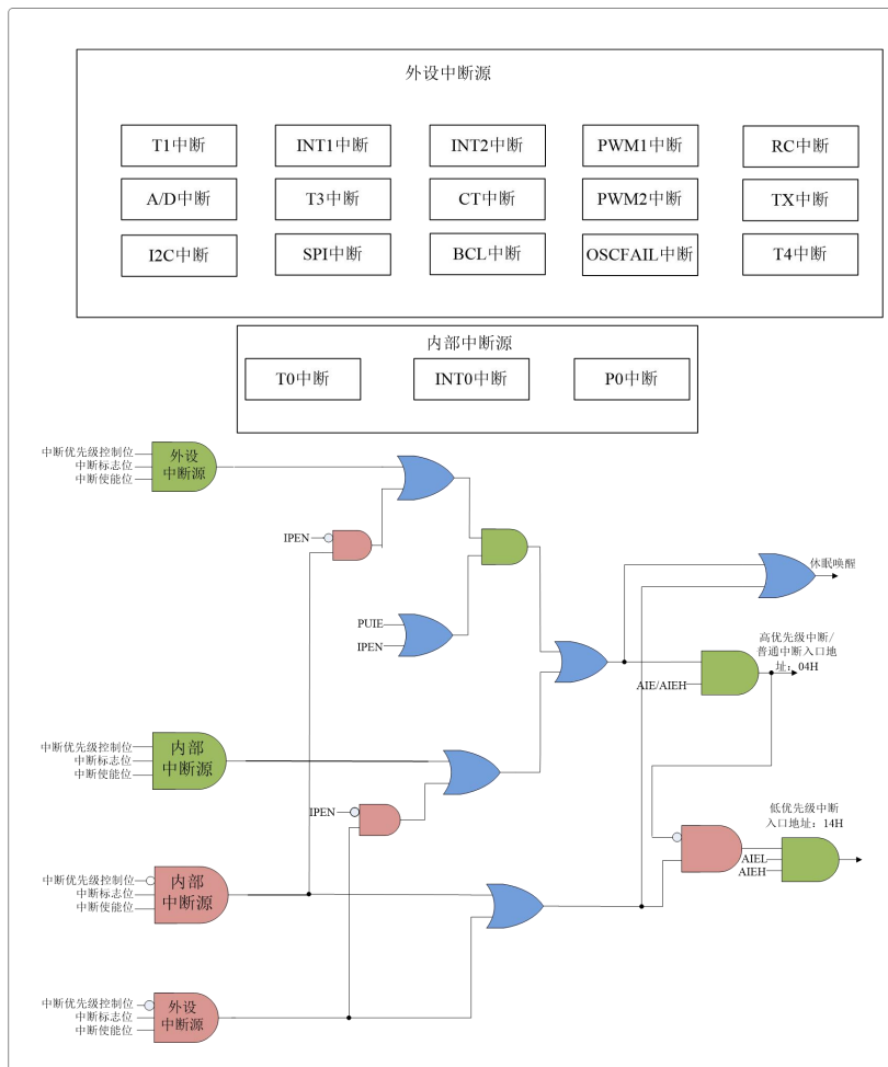
图 5.2 中断逻辑
