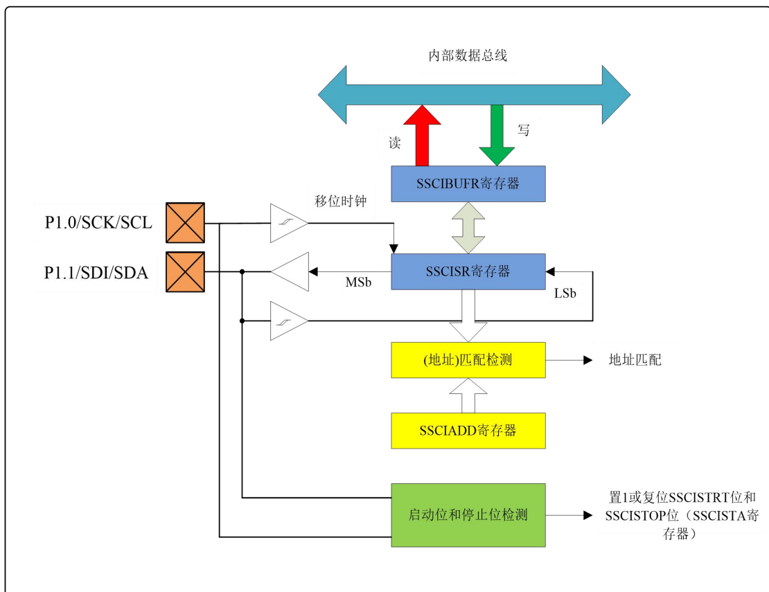
图10.1 I2C模式方框图
