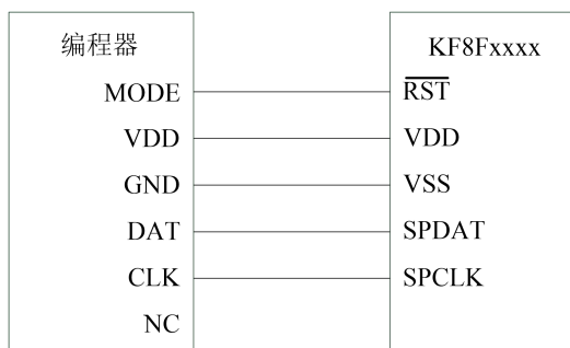
图 1-7 KF8F1000 在线串行编程连接图
