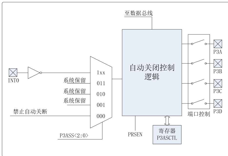
图 7-15 自动关断模式原理框图
