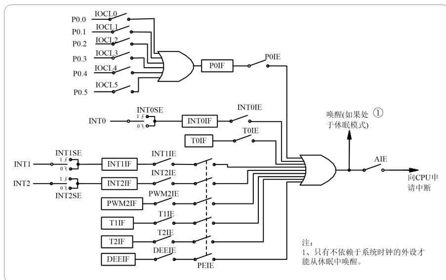
图 5-1 中断逻辑
