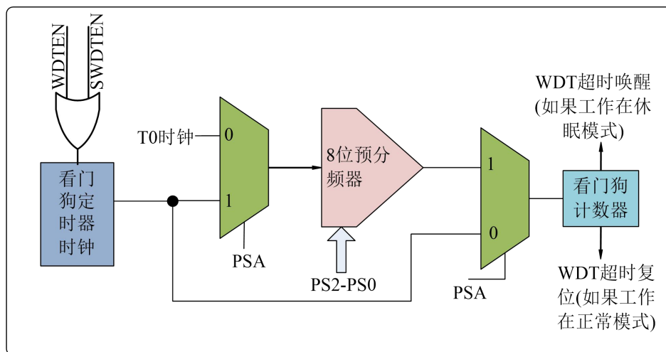
图 10-1 看门狗定时器框图
