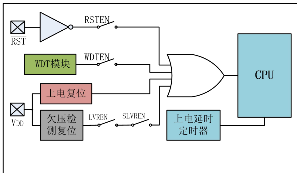
图 8-1 片内复位电路简化框图
