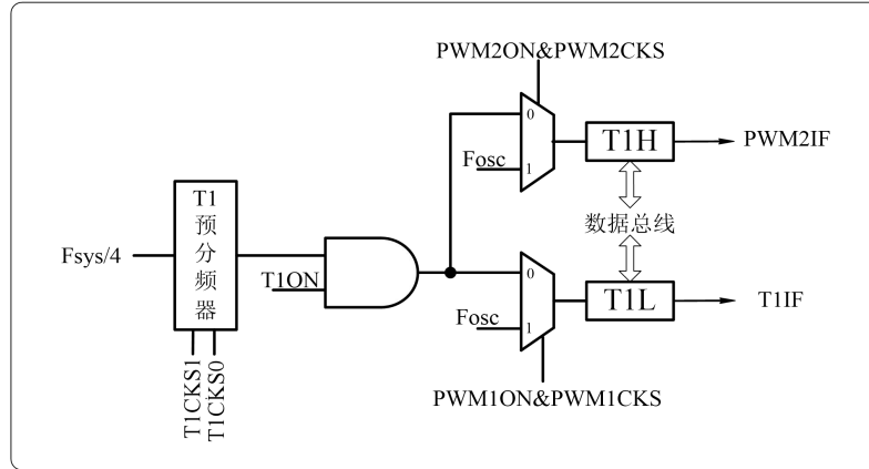
图 7-3 PWM1/2 使能时 T1 时钟源框图
