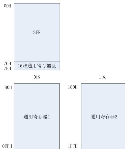
图 3-4 数据存储器地址映射图
