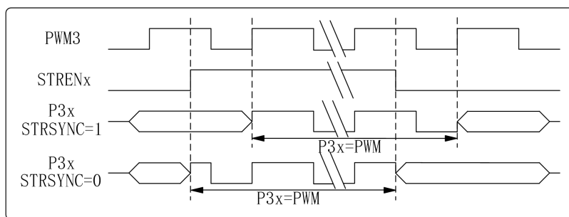
图 7-6 单输出模式 PWM 输出引脚切换
