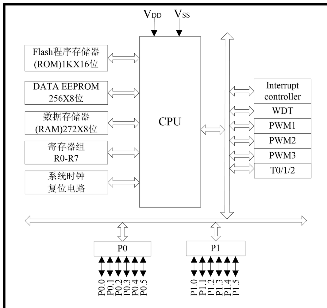
图 1-1 KF8F1000 系统框图
