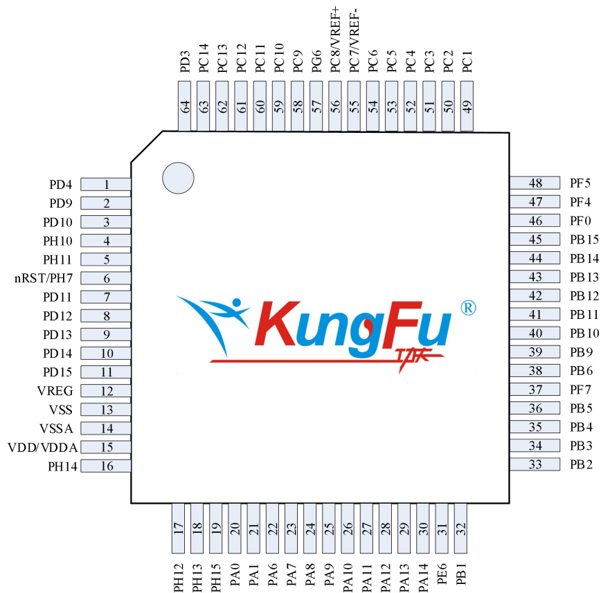
图 2-5 LQFP64
