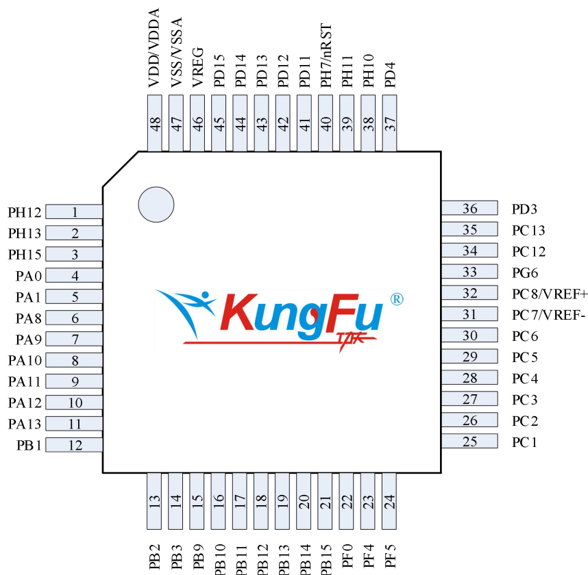
图 2-6 LQFP48
