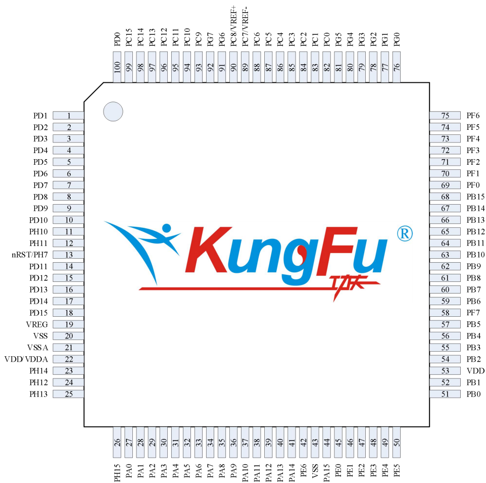
图 2-4 LQFP100
