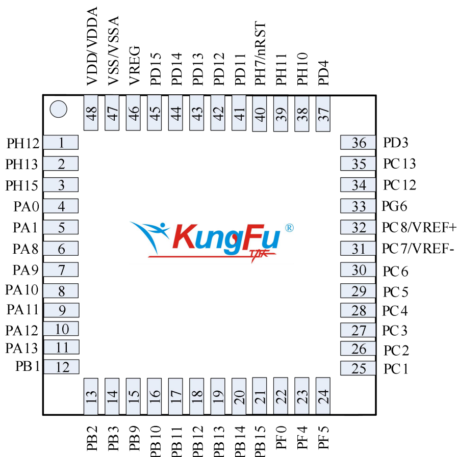
图 2-7 QFN48
