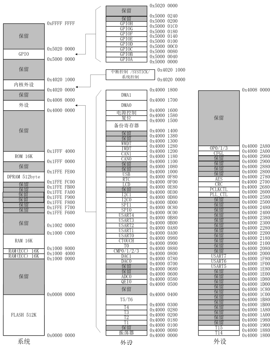
图 4-1 存储空间映射
