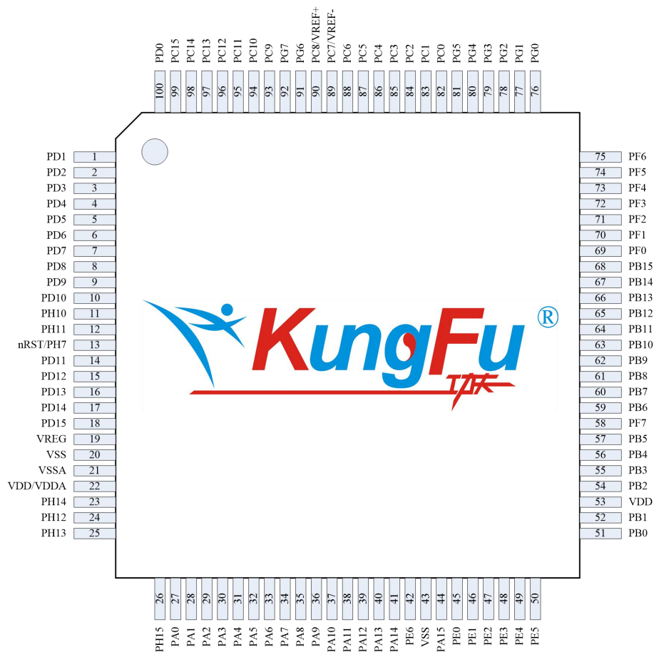
图 2-8 LQFP100
