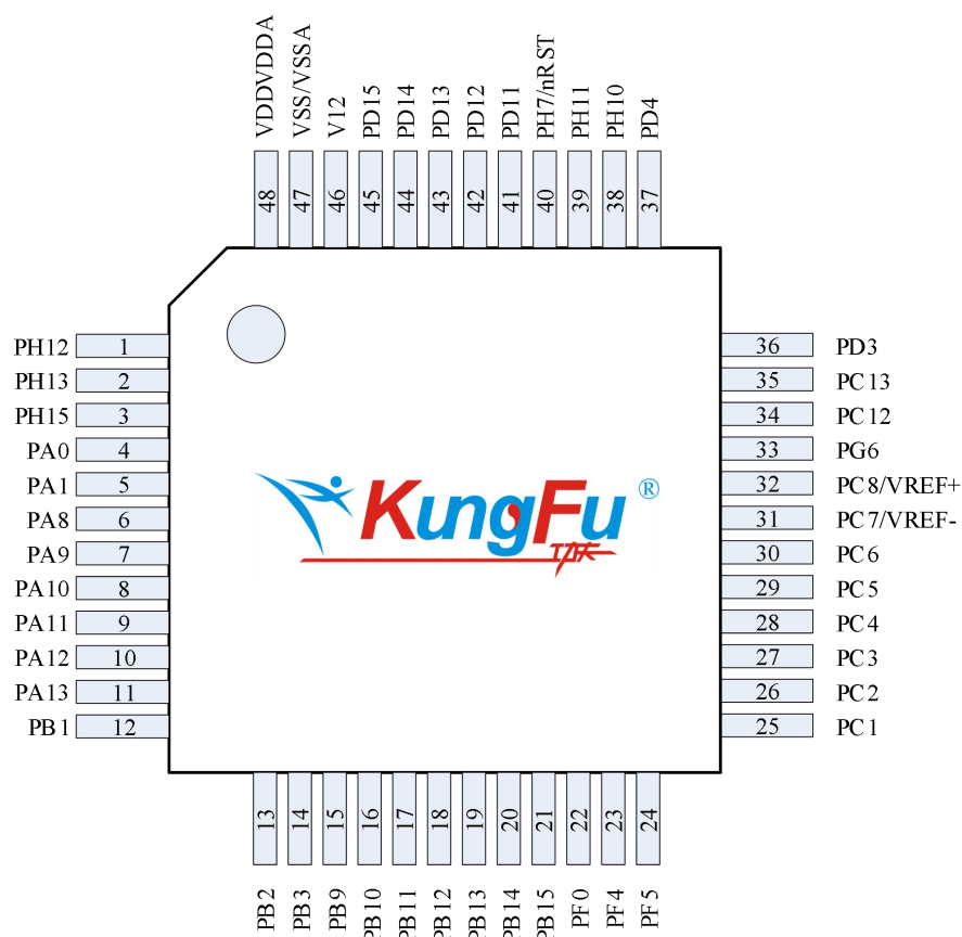
图 2- 6 LQFP48
