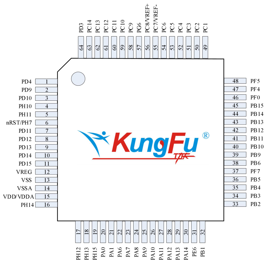
图 2-7 LQFP64
