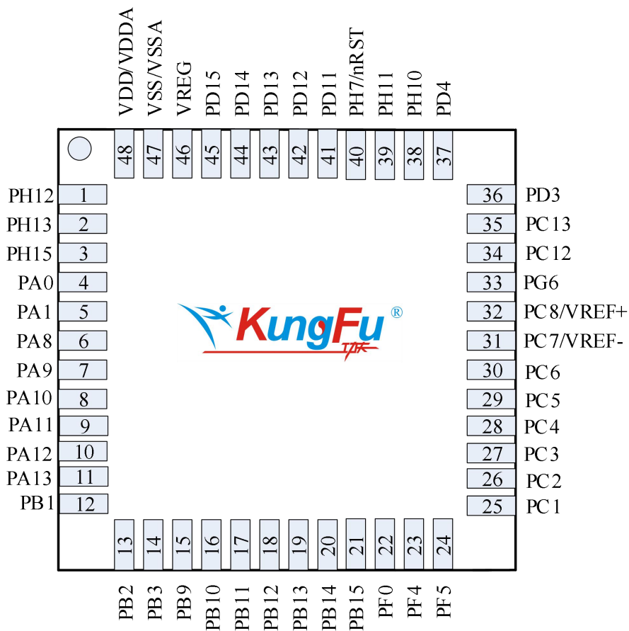
图 2-5 QFN48
