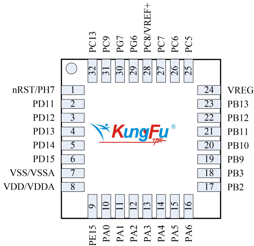
图 2-4 QFN32
