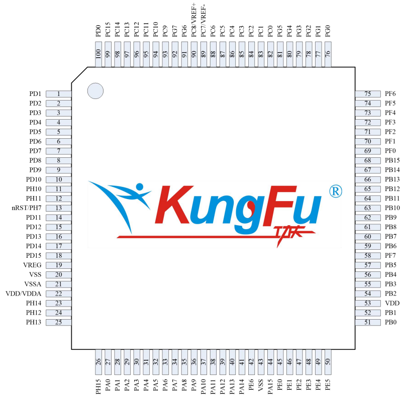
图 2-8 LQFP100
