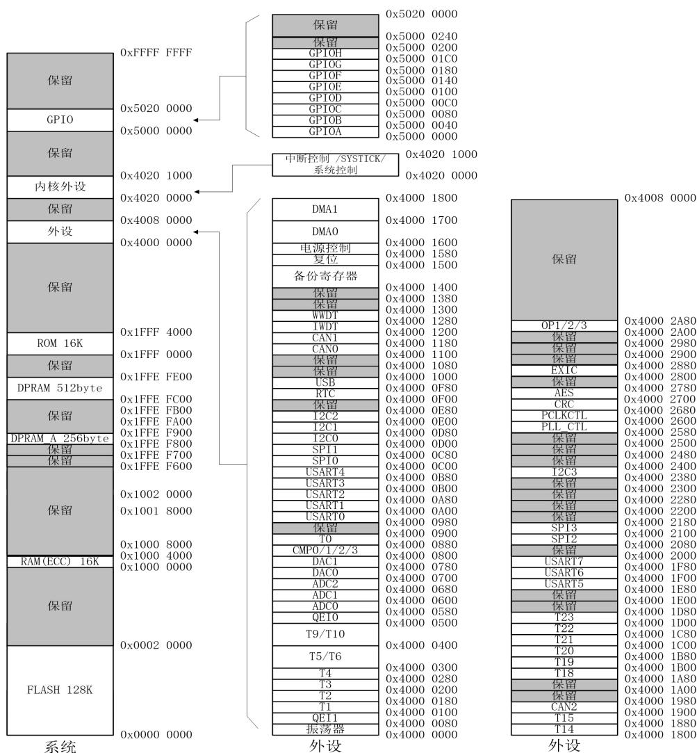
图 4-1 存储空间映
