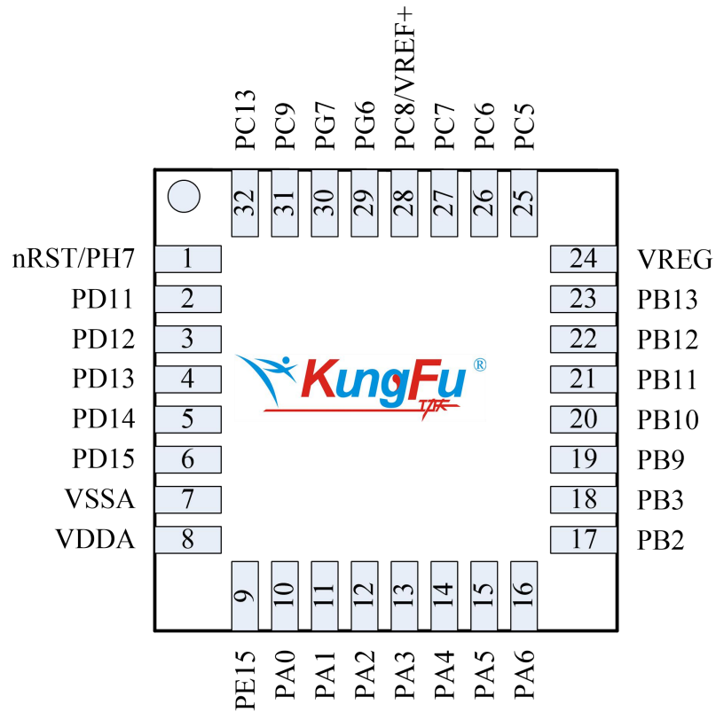
图 2-4 QFN32
