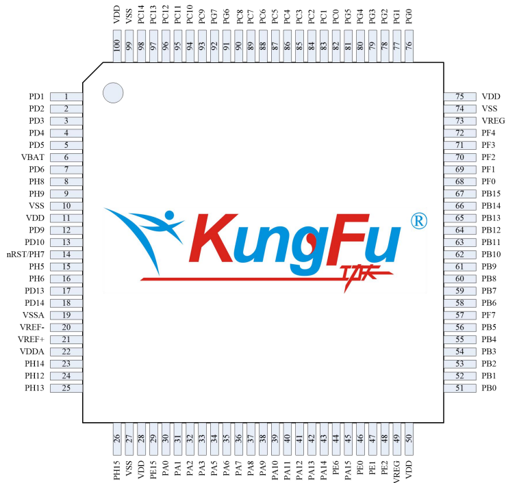
图 2-4 LQFP100
