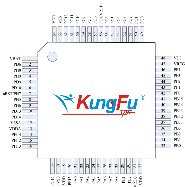
图 2-5 LQFP64
