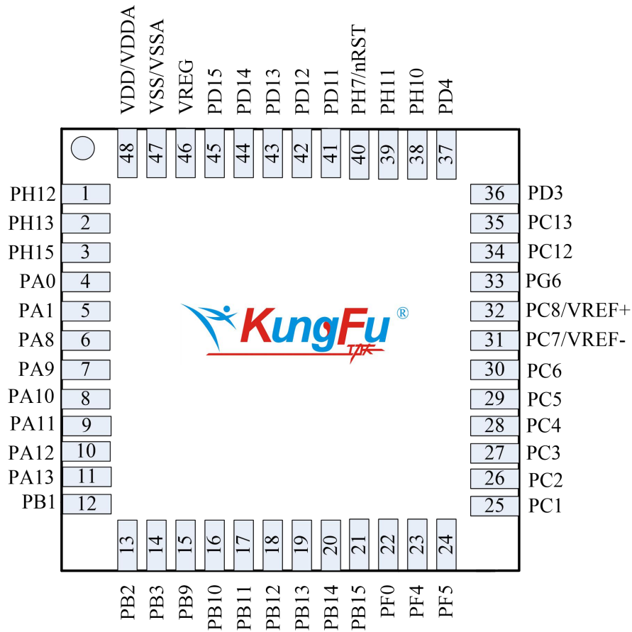
图 2-7 QFN48
