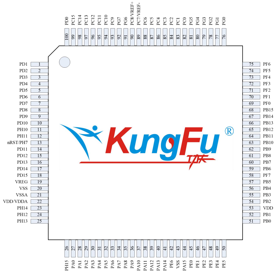
图 2-4 LQFP100
