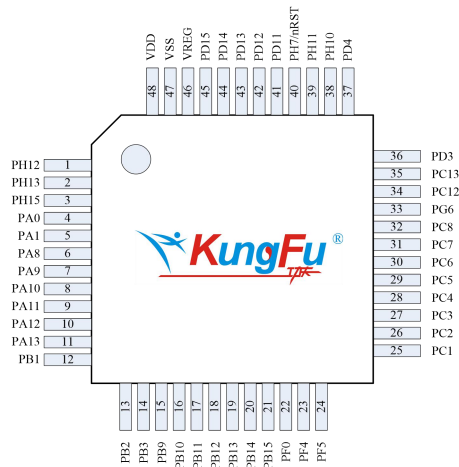
图 2- 5 LQFP48
