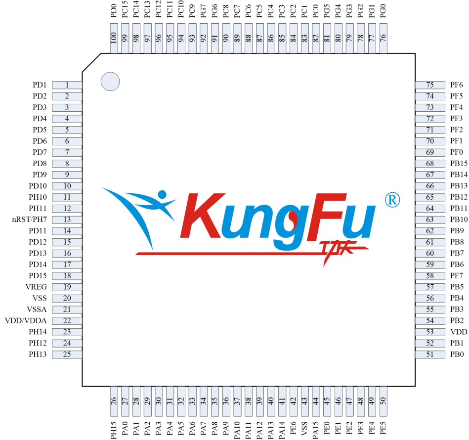
图 2-3 LQFP100
