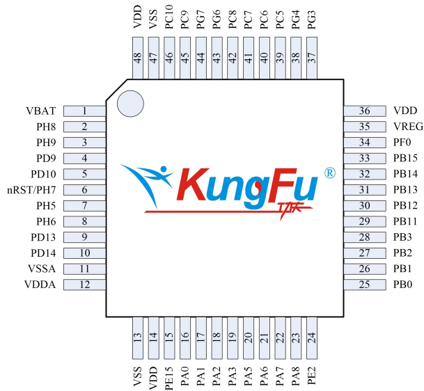
图 2-4 LQFP48
