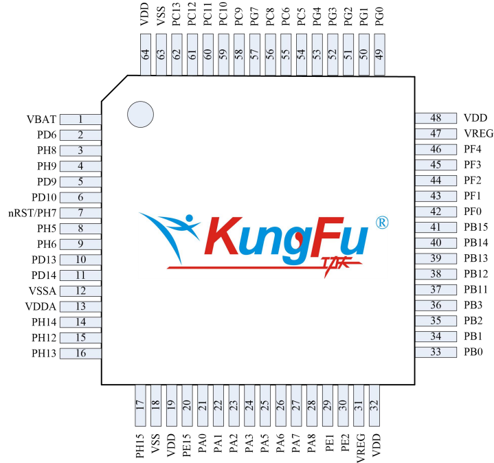
图 2-3 LQFP64
