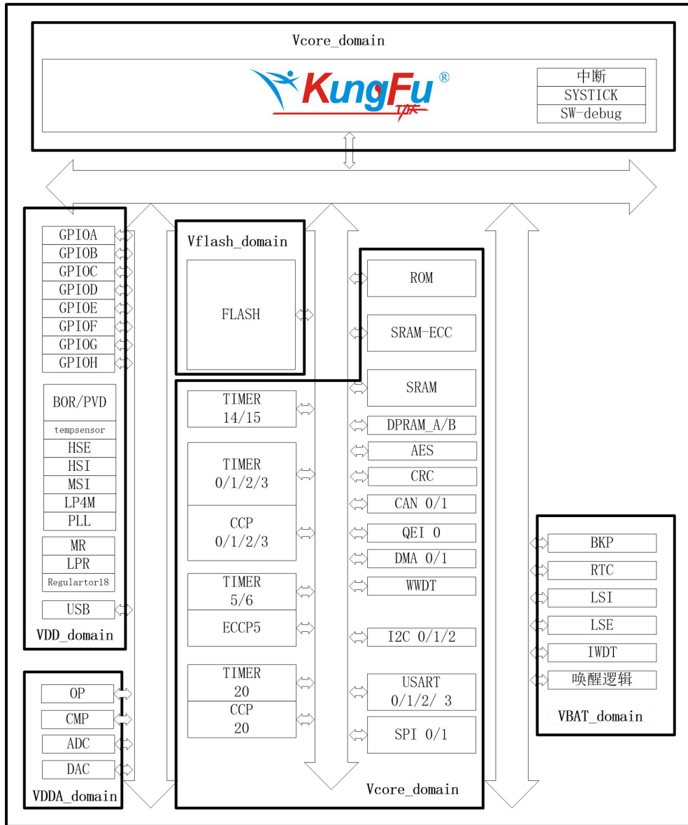
图 2-2 系统结构框图
