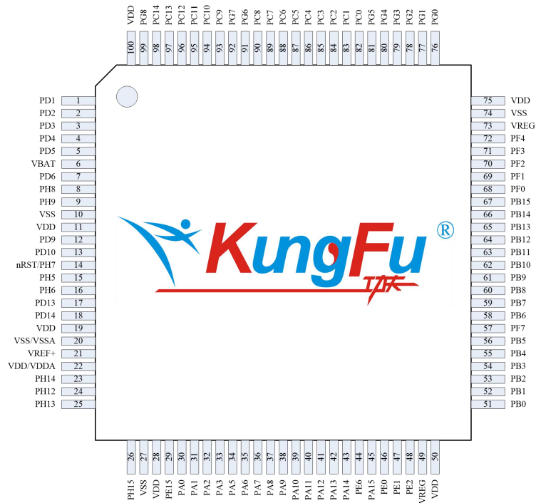
图 2-3 LQFP100
