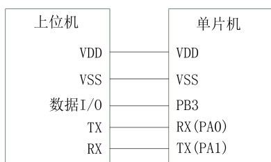
图 2-1 ISP 模式编程接口
