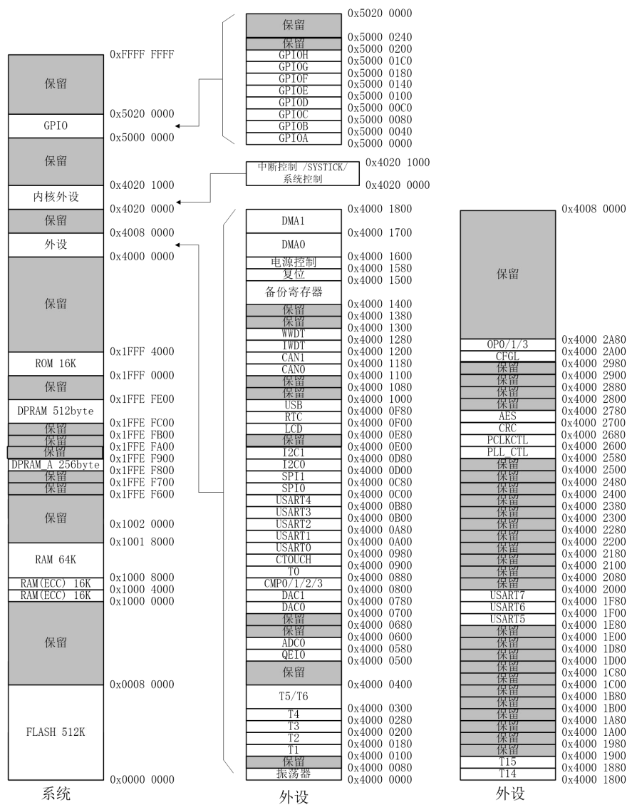
图 4-1 存储空间映
