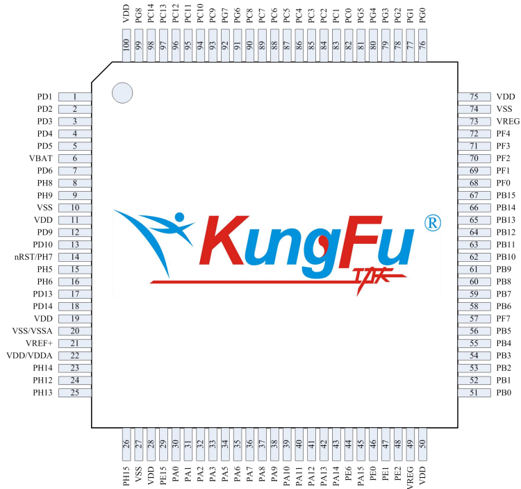
图 2-2 LQFP100
