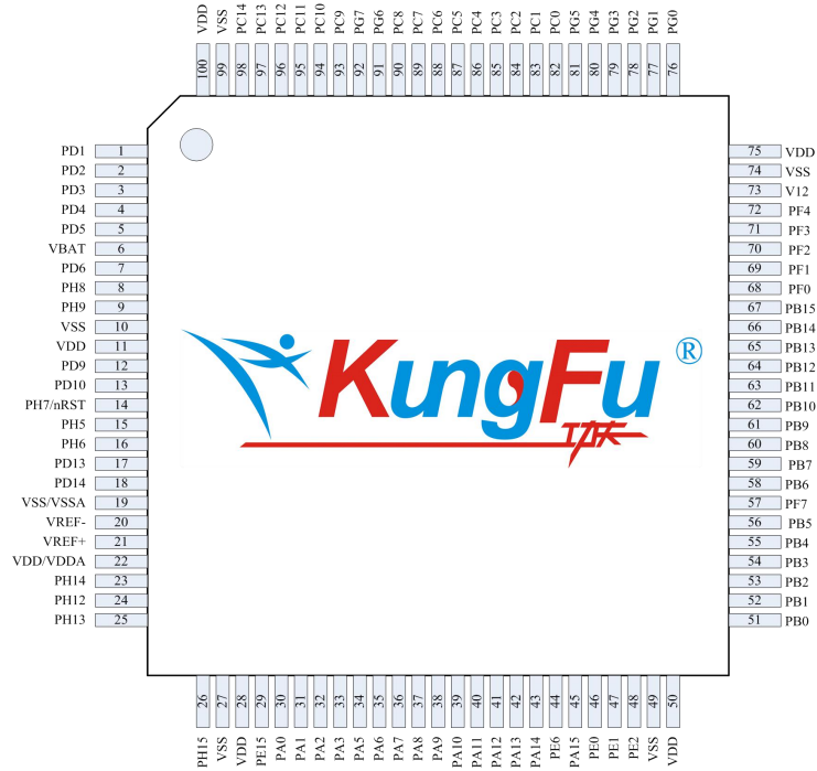
图 2-2 LQFP100
