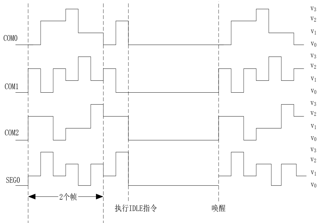
图 16.16 当 \overline{\text{SLPEN}} = 1 是进入/退出休眠模式
