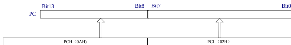
图 3.4 PCL/PCH 寄存器的使用
