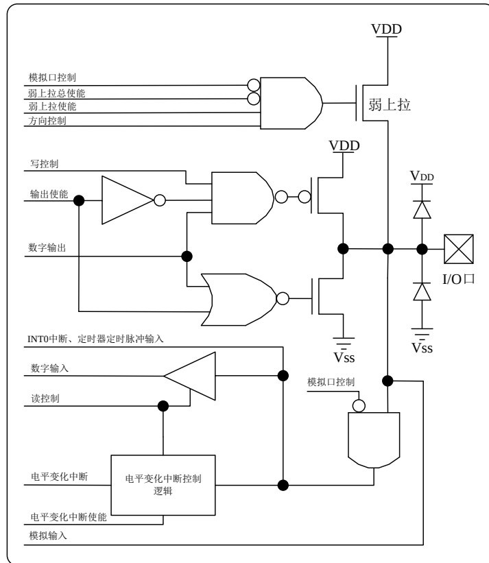
图 2.3.1 P0.0~P0.2、P0.7 口引脚内部原理框图
