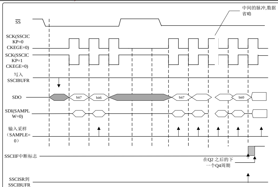
图13.31 从动时序图
