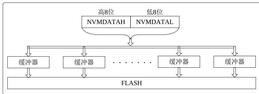
图 3.8 写操作
