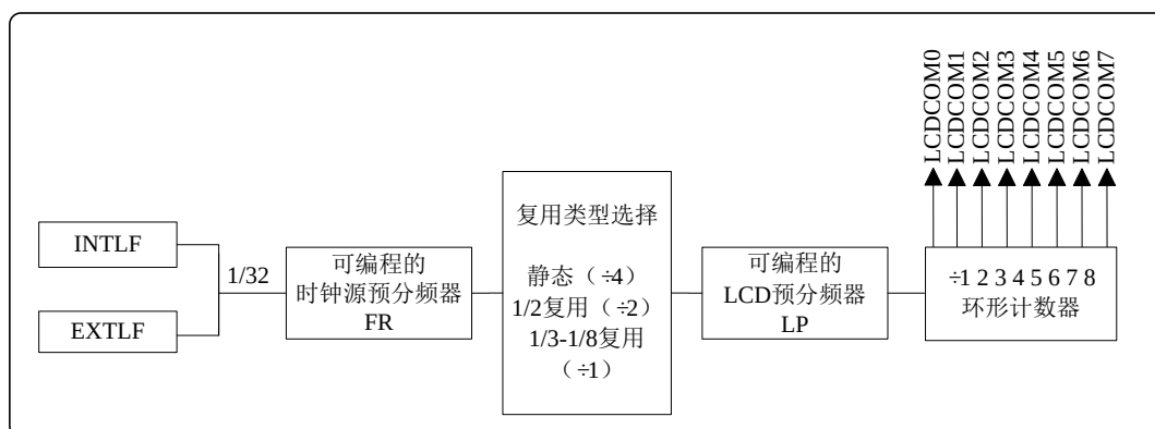
图 16.2 LCD 预分频器图
