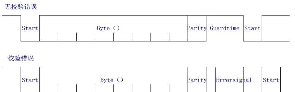
图 14.18 7816 接口时序
