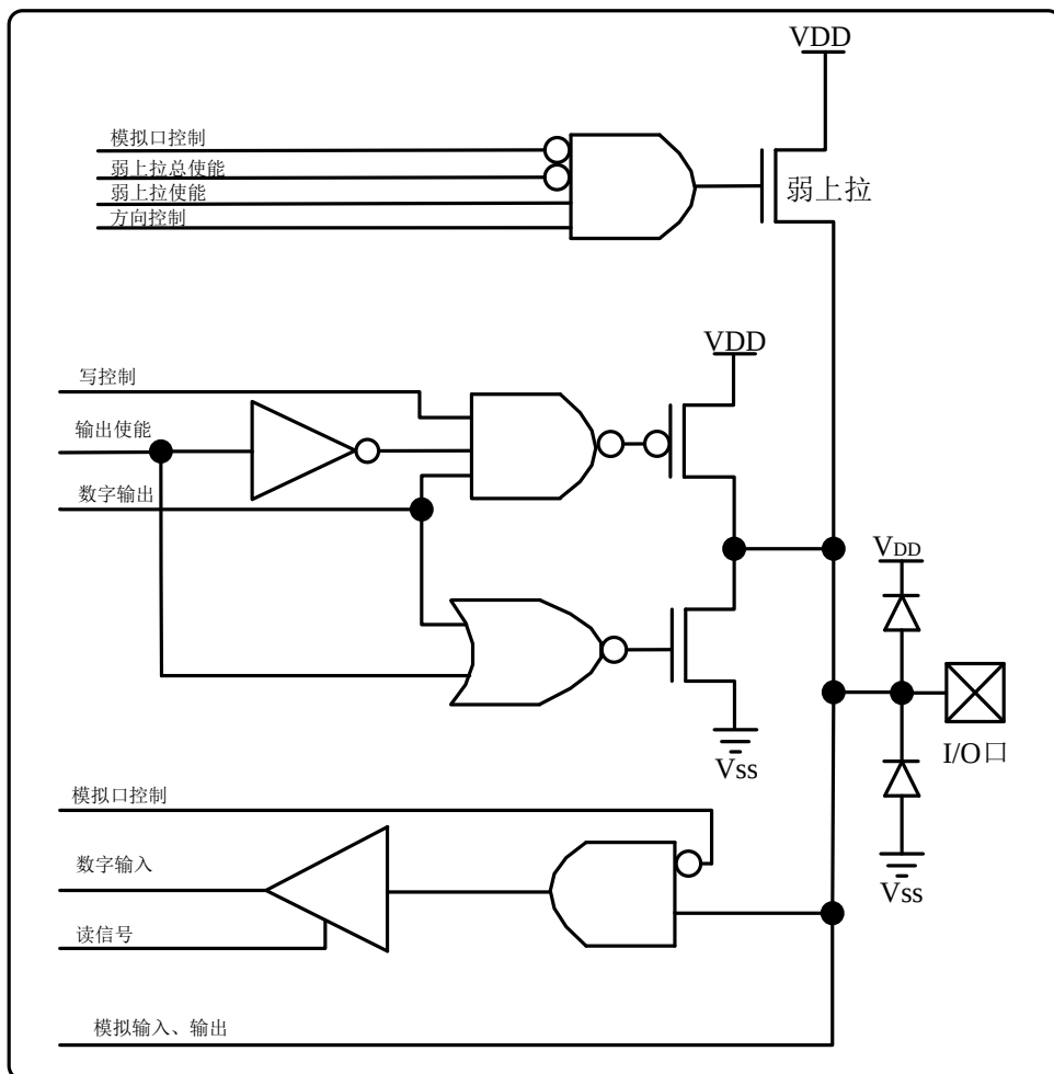
图 2.10 P7 口引脚原理功能框图
