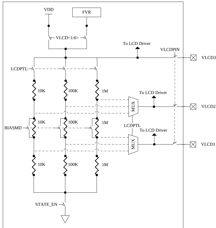
图 16.3 LCD 偏置电路原理框图
