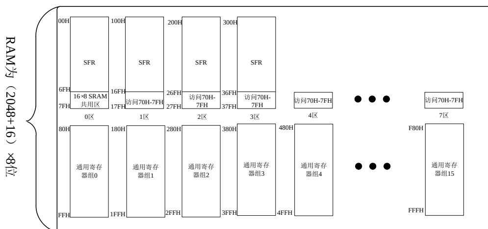
图 3.6 数据存储区地址映射图
