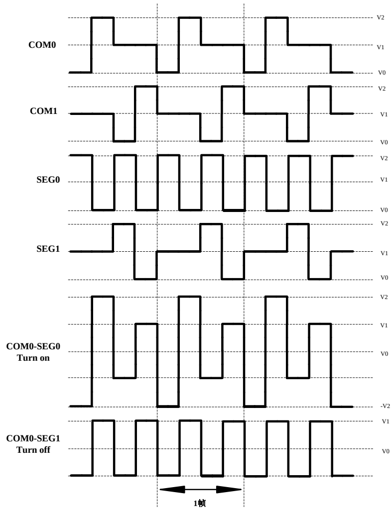
图 16.5 在 1/2 复用、1/2 偏置驱动时的 A 型波形
