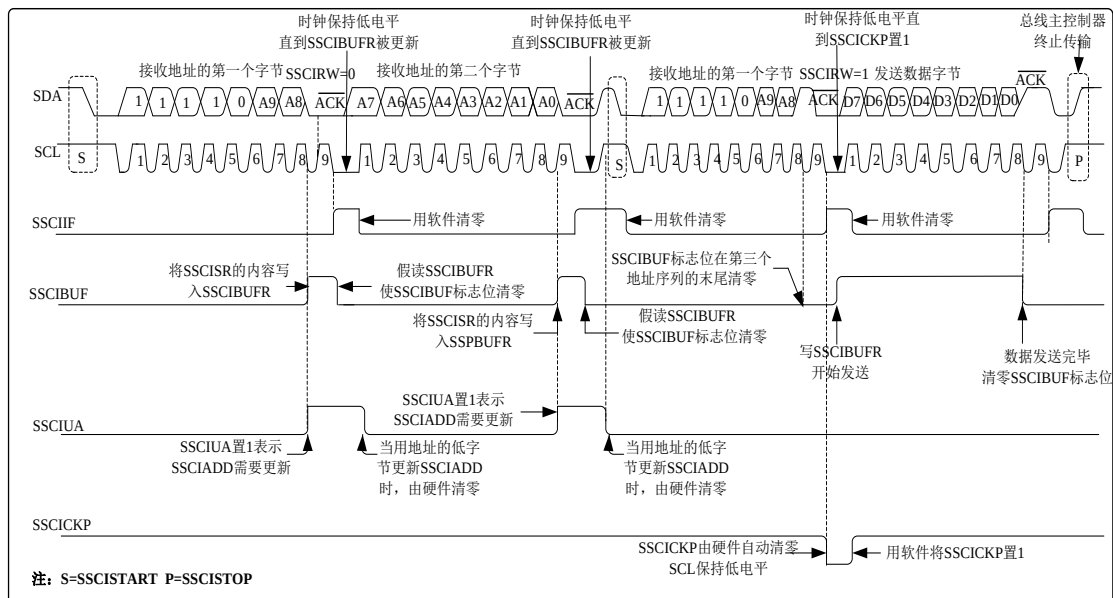
图 13.5 从动模式时序（发送，10 位地址）
