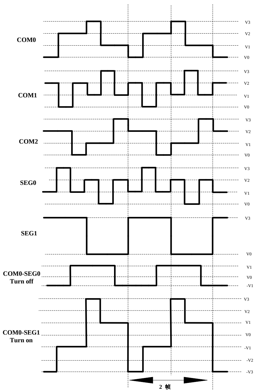
图 16.12 在 1/3 复用、1/3 偏置驱动时的 B 型波形
