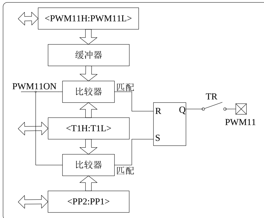
图 9.1 PWM11 逻辑框图
