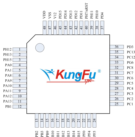
图 2-4 LQFP48
