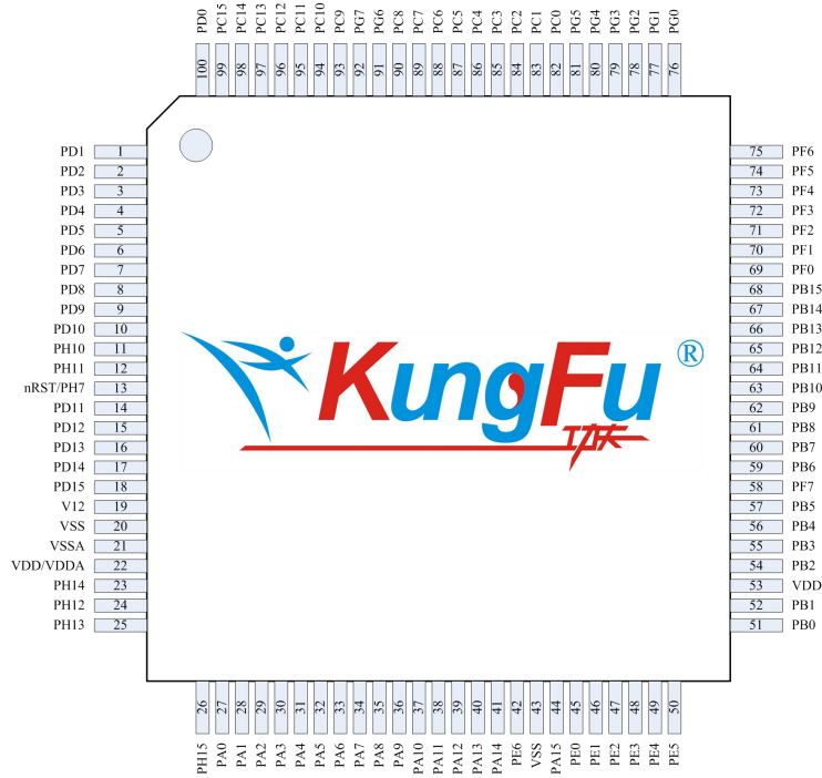
图 2-2 LQFP100
