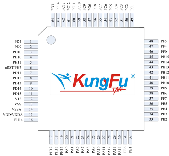
图 2-3 LQFP64
