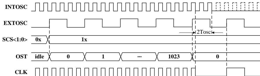
图 1.8 切换至外部时钟源时时钟信号同步时序图
