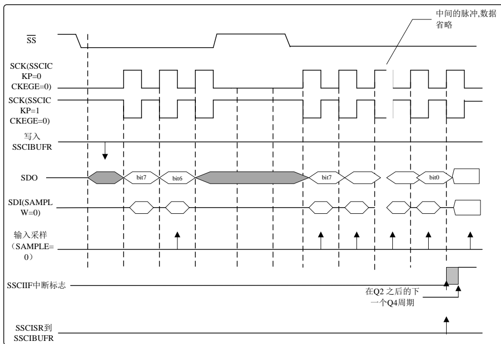
图10.31 从动时序图
