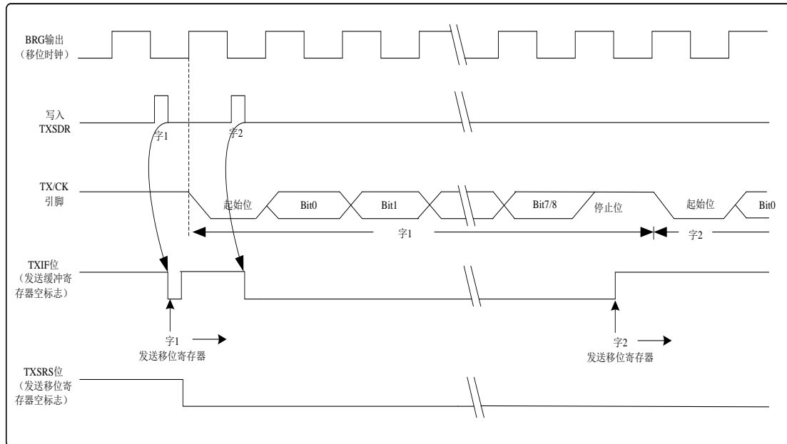
图 11.10 全双工异步发送（一字符接一字符）
