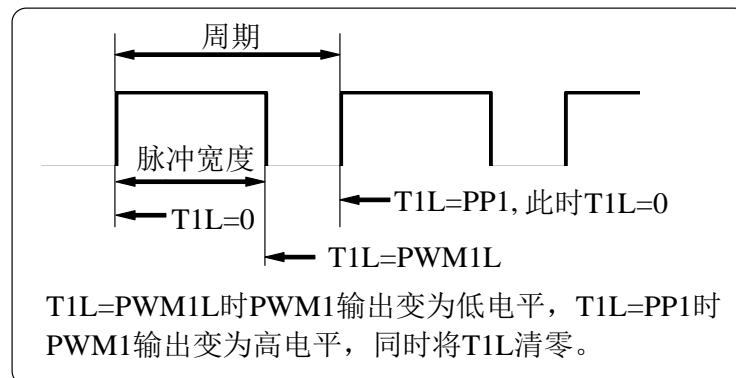
图 8.2 PWM1 输出波形图
