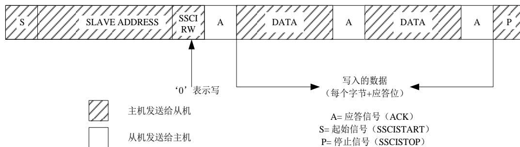
图 10.13 I2C 协议典型写数据帧格式
