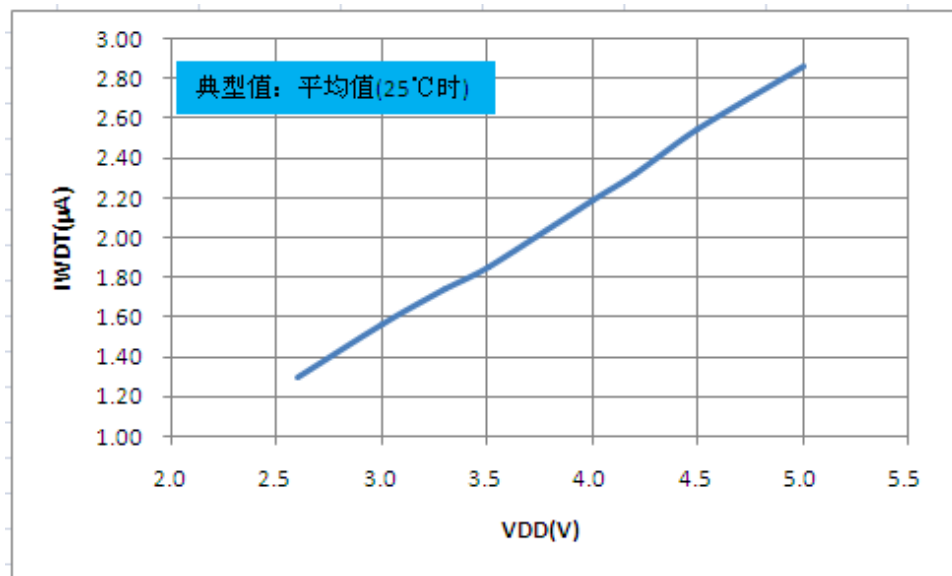
图20.4: 看门狗电流 - VDD关系曲线图
