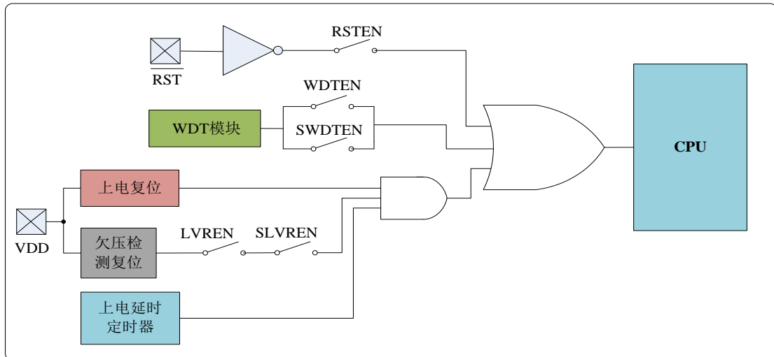
图 16.1 片内复位电路简化框图
