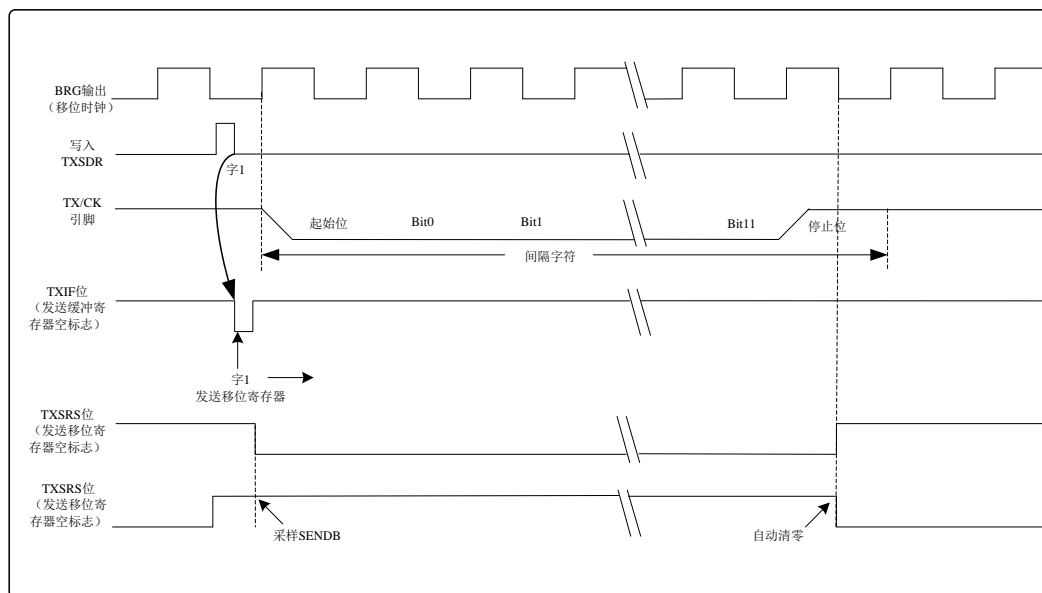
图 11.6 发送间隔字符时序
