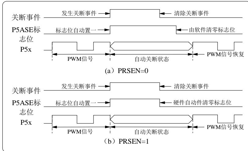
图 9.20 自动重启和软件重启 PWM
