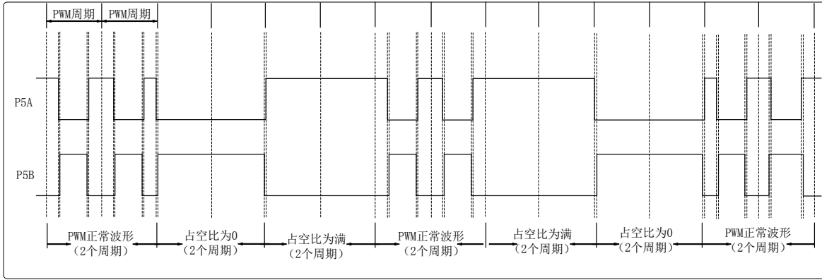
图 9.13 切换电平示意图（中心对齐模式下）
