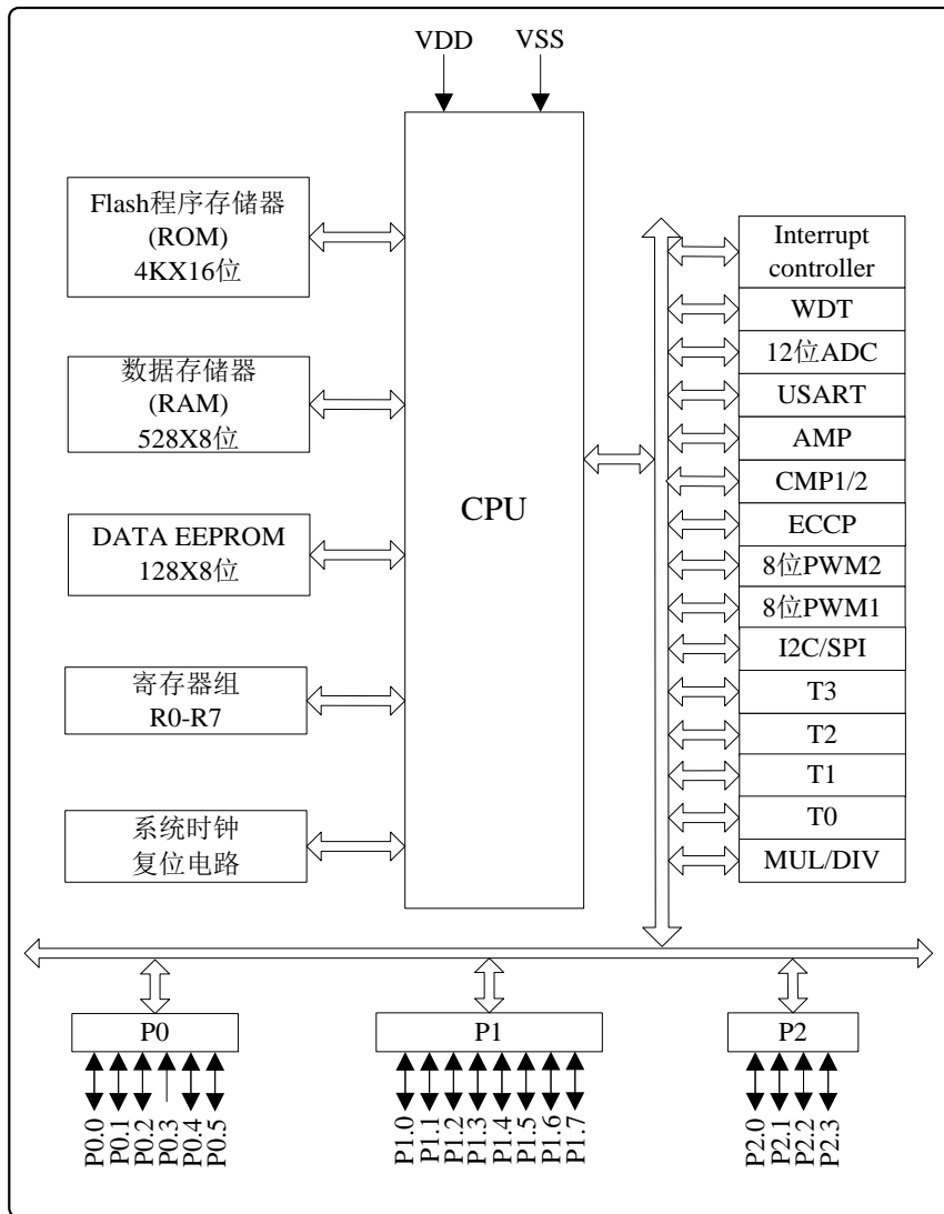
图 1.1b KF8F3112/22/32 系统框图
