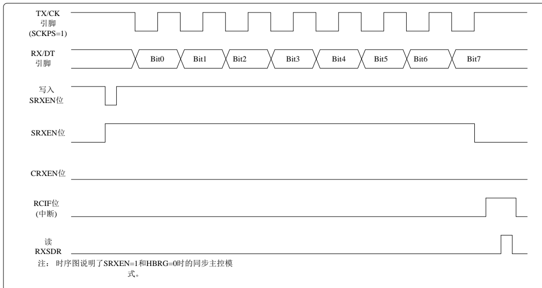
图 11.16 半双工同步接收（主控模式，SRXEN=1，SCKPS=1）
