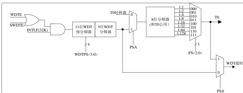
图 18.1 看门狗定时器框图
