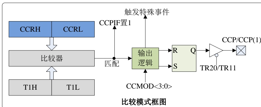
图9.2 比较模式原理框图
