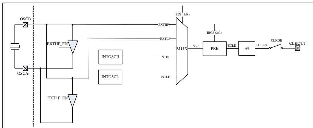
图 1.3 时钟模块原理框图
