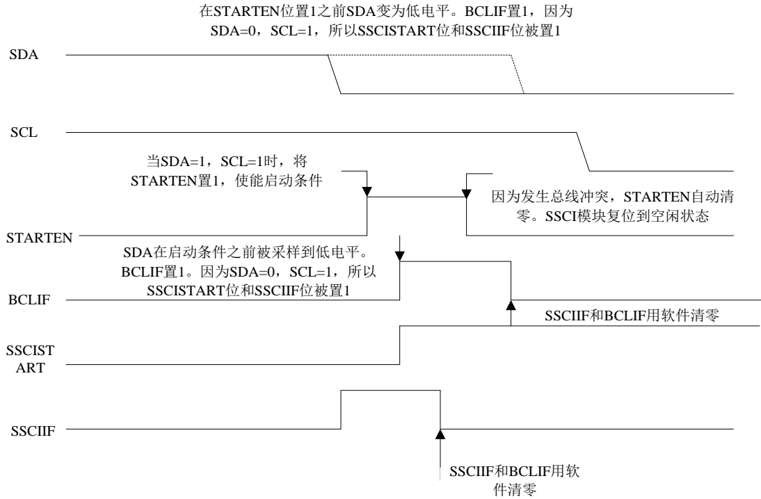
图10.21 启动条件期间的总线冲突（仅SDA）
