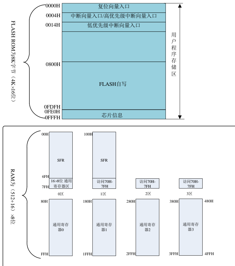
图 3.1 KF8F3110/12/20/22/30/32 存储器组织图
