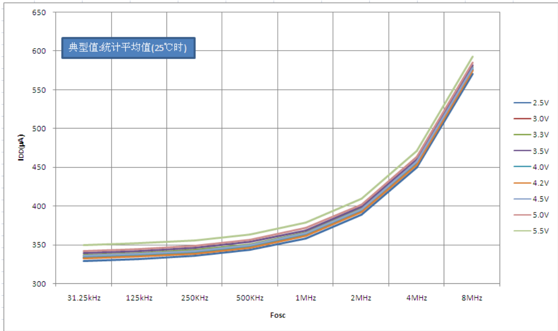
图20.1c: 不同VDD时KF8F3120/22典型IDD — Fosc 关系曲线图
