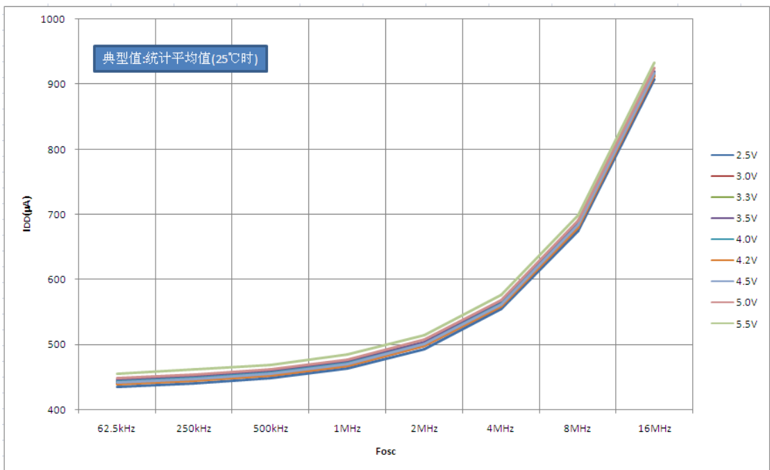
图20.1d: 不同VDD时KF8F3130/32典型IDD — Fosc 关系曲线图
