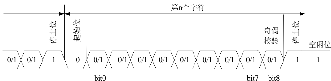
图 11.7 全双工异步通信数据结构图
