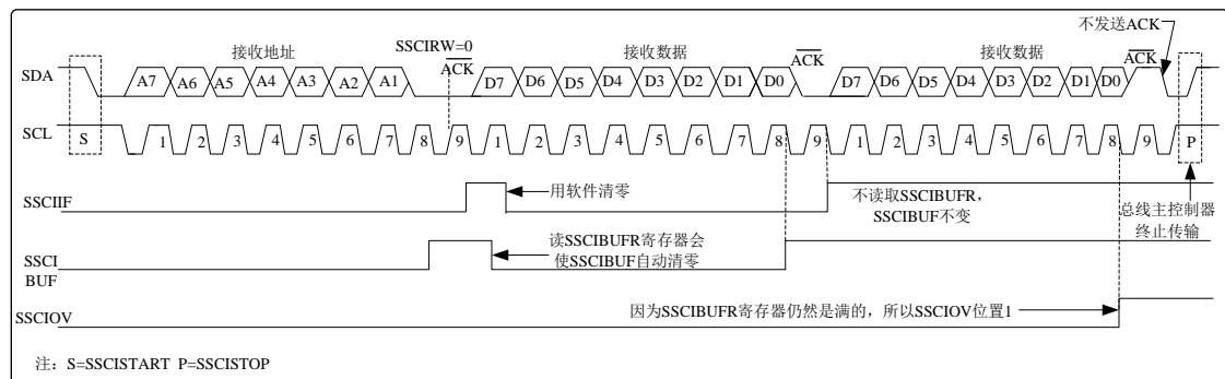
图10.2 从动模式时序（接收，7位地址）
