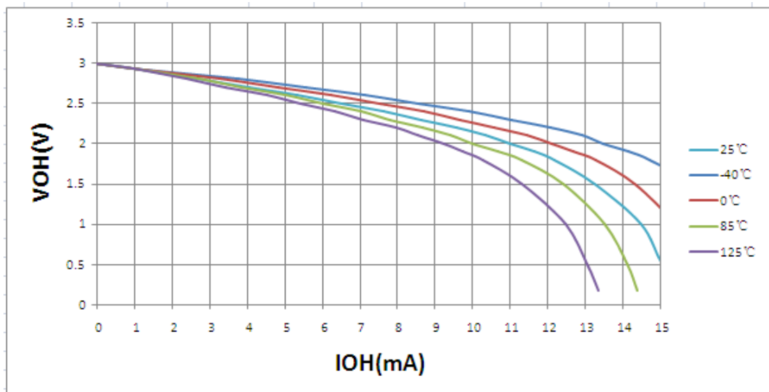
图20.7: 不同温度时 V_{OH} — I_{OH} 关系曲线图 ( V_{DD} = 3.0V )
