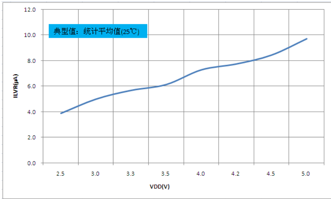
图 20.5: 欠压检测复位电流 I_{LVR} - VDD 关系曲线图
