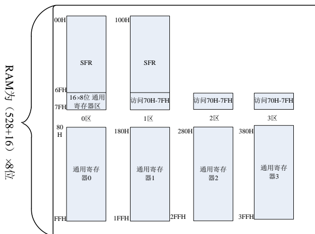
图 3.5 数据存储器地址映射图
