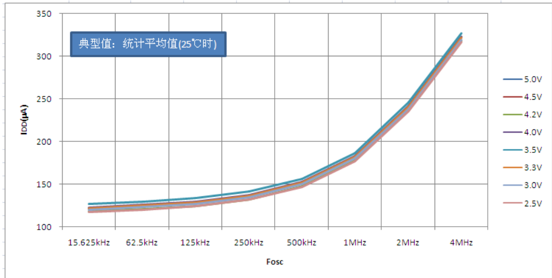
图20.1a: 不同VDD时KF8F3110典型 I_{DD} — F_{osc} 关系曲线图
