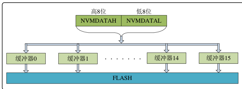
图 3.7 FLASH 写操作
