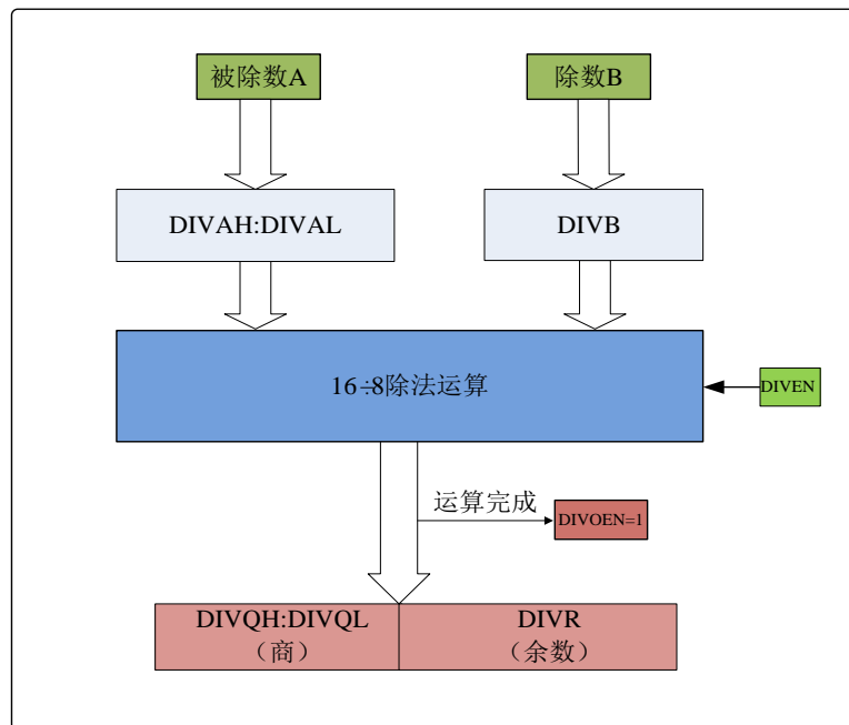
图 15.1 硬件除法器原理框图
