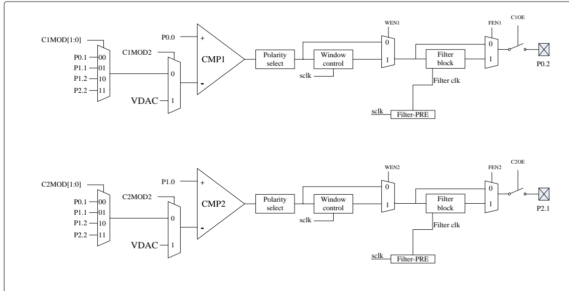
图 13.1 模拟比较器原理框图
