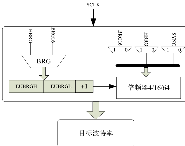
图 11.2 USART 目标波特率产生原理框图
