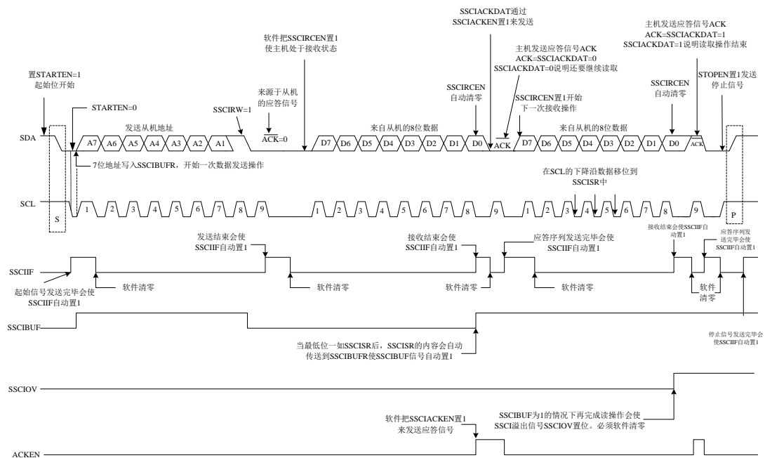
图10.16 I2C主控模式接收数据时序图（7位地址）
