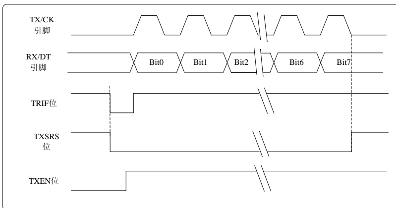
图 11.14 半双工同步发送（通过 TXEN）
