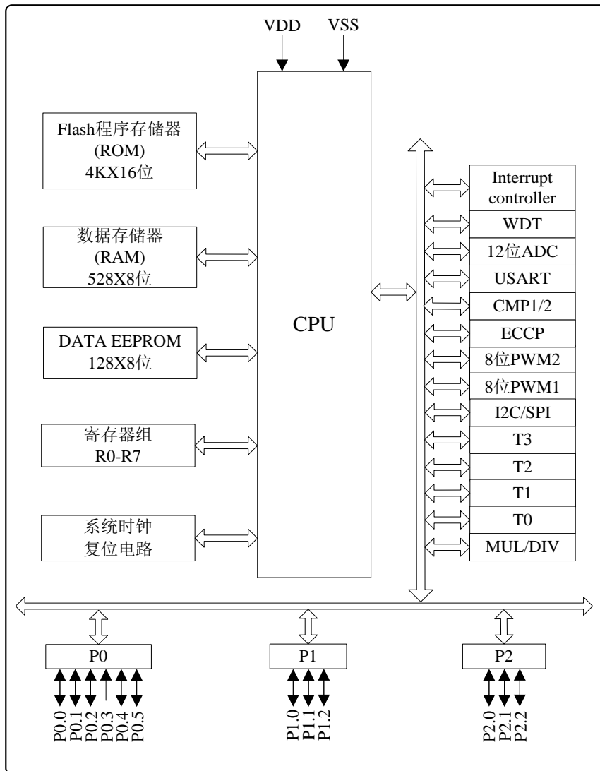
图 1.1a KF8F3110/20/30 系统框图
