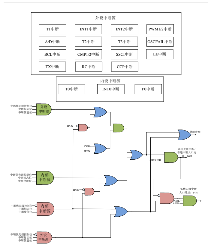
图 5.2 中断逻辑
