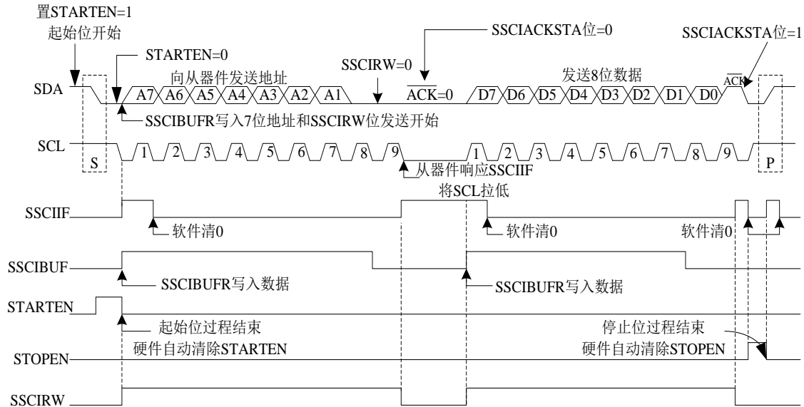
图 10.14 硬件 I2C 主控模式发送数据时序图（7 位地址）
