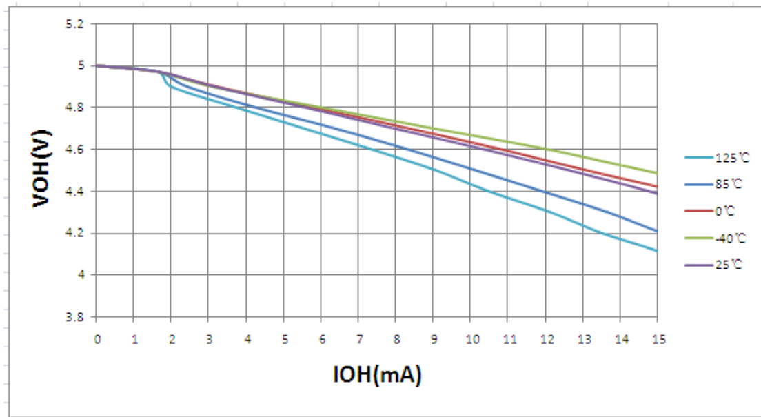
图20.6: 不同温度时 V_{OH} — I_{OH} 关系曲线图 ( V_{DD} = 5.0V )
