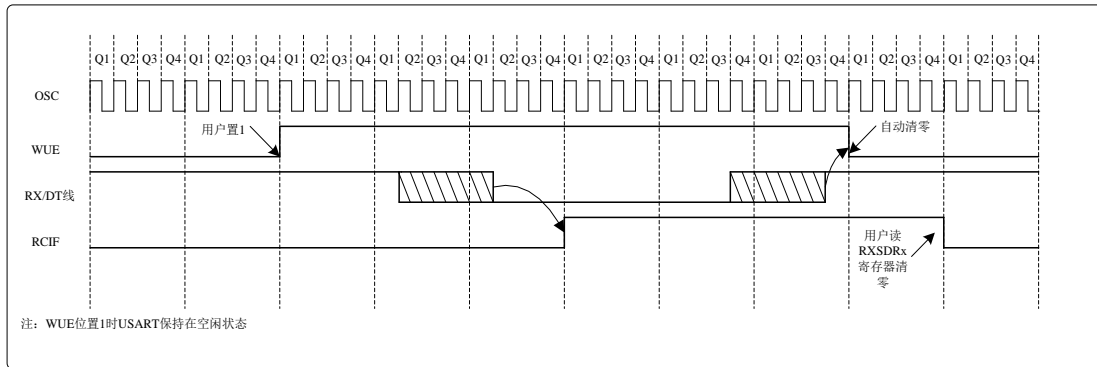
图 11.4 正常工作下的自动唤醒时序
