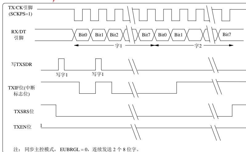
图 11.13 半双工同步发送(SCKPS=1)
