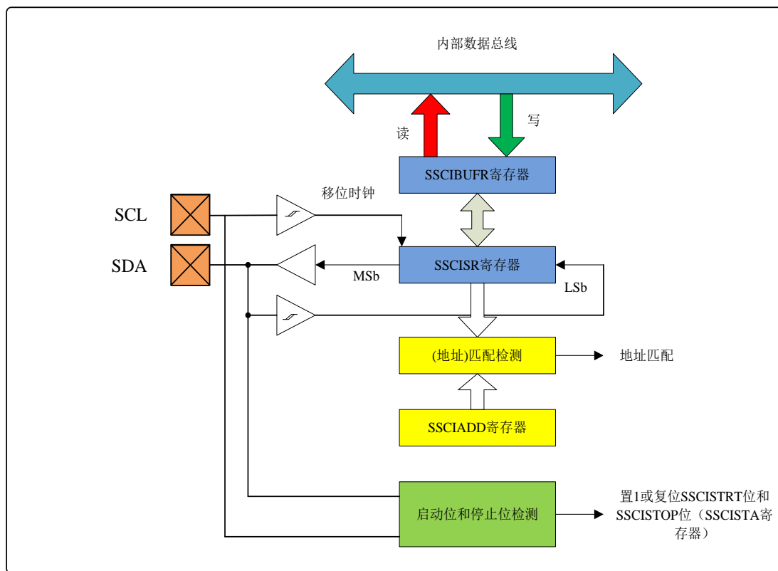
图10.1 I2C模式方框图
