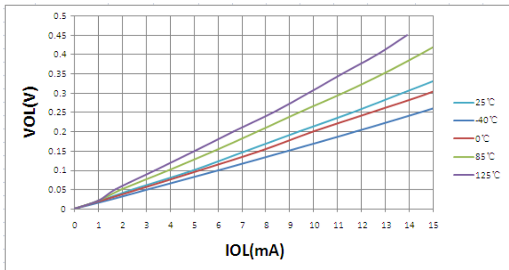
图20.9: 不同温度时VOL — IOL 关系曲线图 (VDD = 3.0V)
