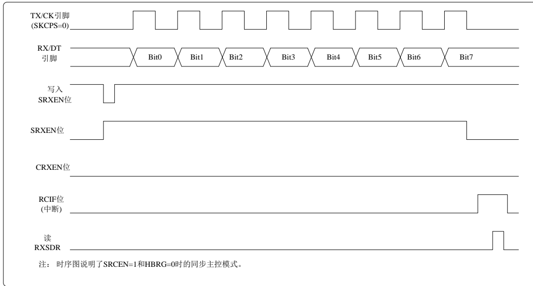
图 11.15 半双工同步接收（主控模式，SRXEN=1，SCKPS=0）
