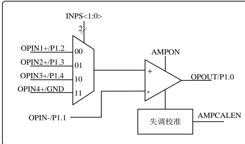
图 12.1 运放内部框图
