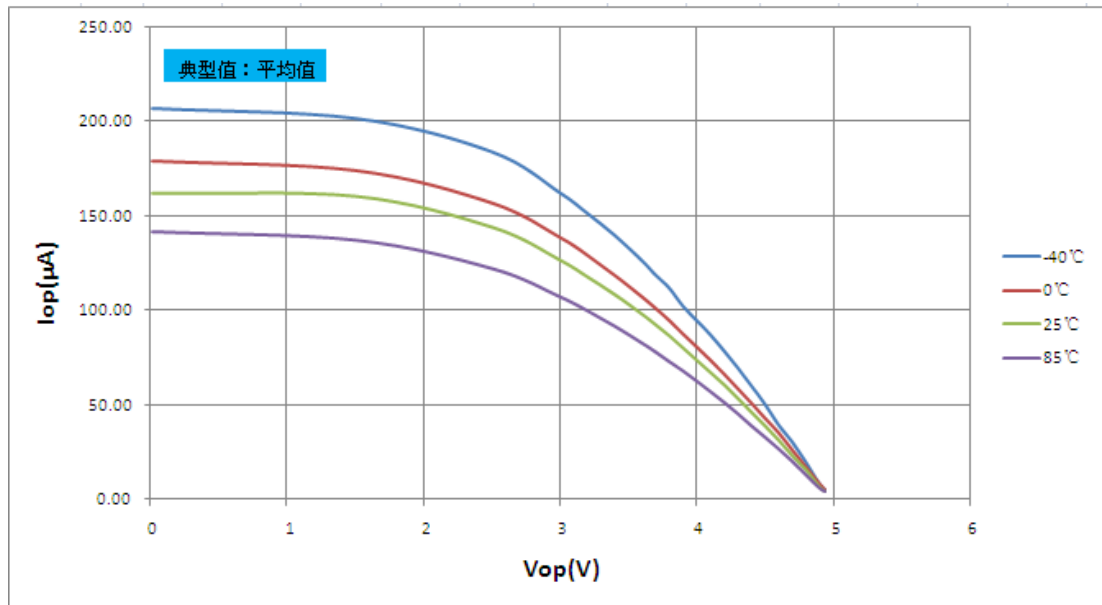
图20.10: 不同温度时VOP—IOP 关系曲线图 (VDD =5.0V)
