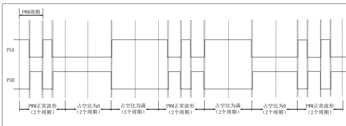
图 9.12 切换电平示意图（边沿对齐模式下）
