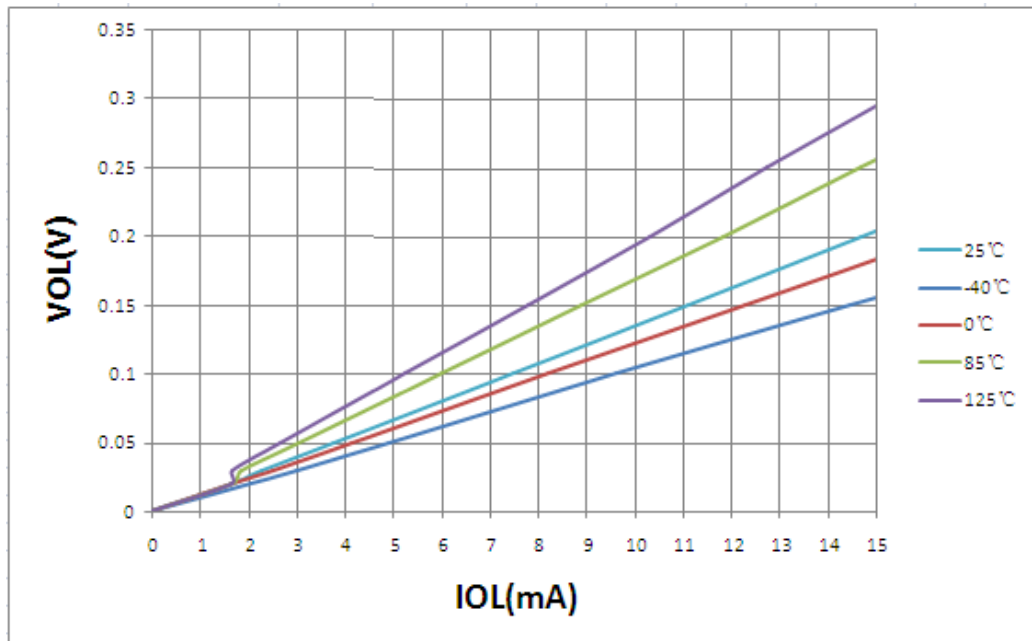
图20.8: 不同温度时VOL — IOL 关系曲线图 (VDD = 5.0V)
