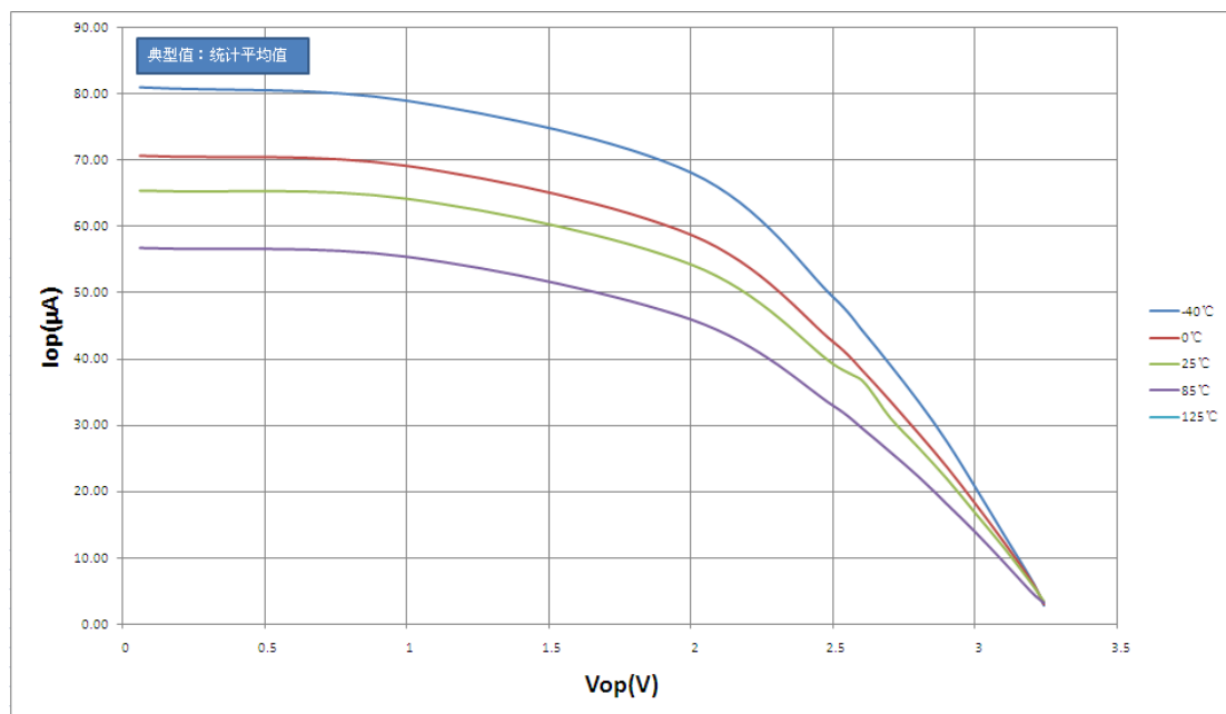
图 20.11: 不同温度时 VOP—IOP 关系曲线图 (VDD =3.3V)
