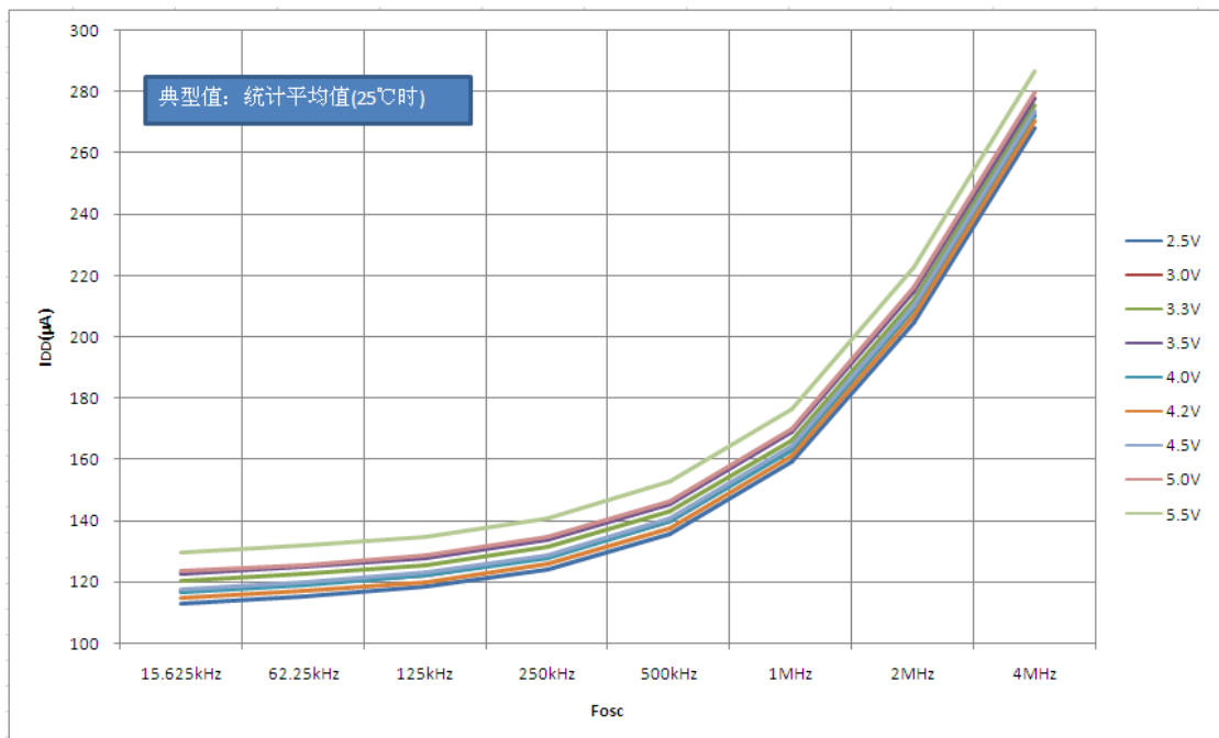
图20.1b: 不同VDD时KF8F3112典型 I_{DD} — F_{osc} 关系曲线图
