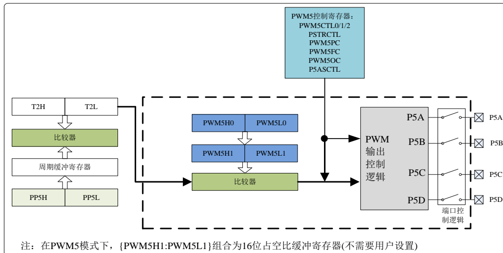
图 9.3 PWM5 原理框图
