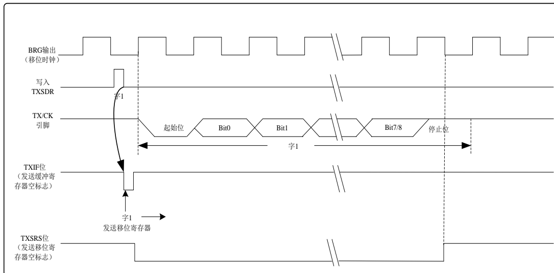
图 11.9 全双工异步发送（两字符间有空闲位）
