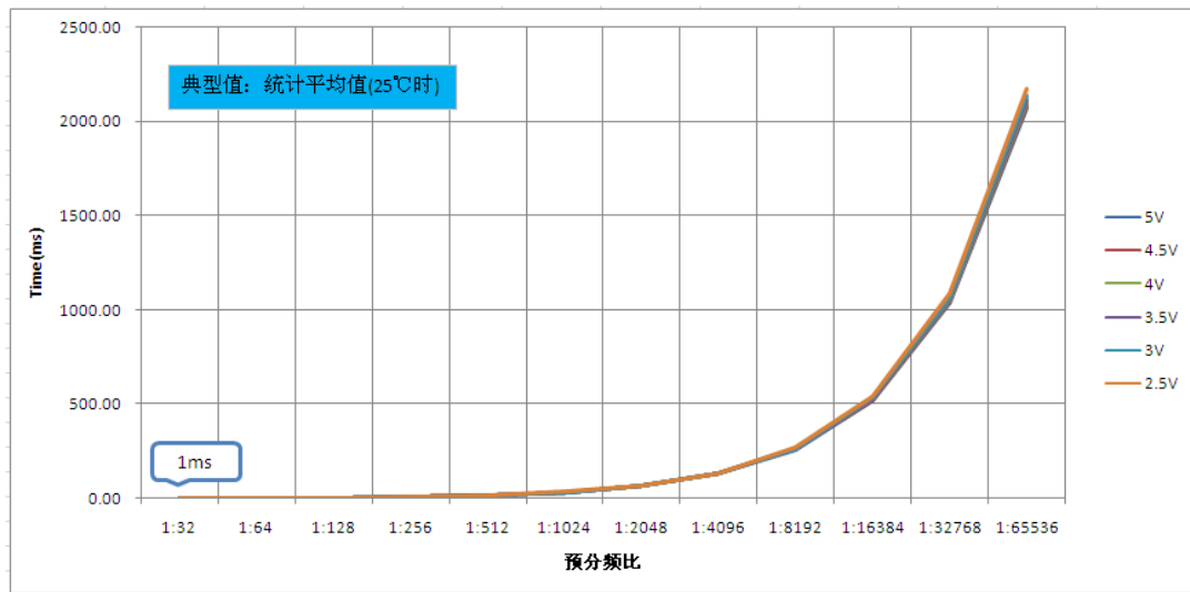
图20.3: 不同VDD时看门狗预分频比 - 周期关系曲线图
