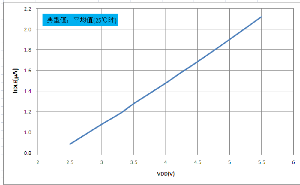
图 20.2: 不同 VDD 时典型 IDLE - VDD 关系曲线图
