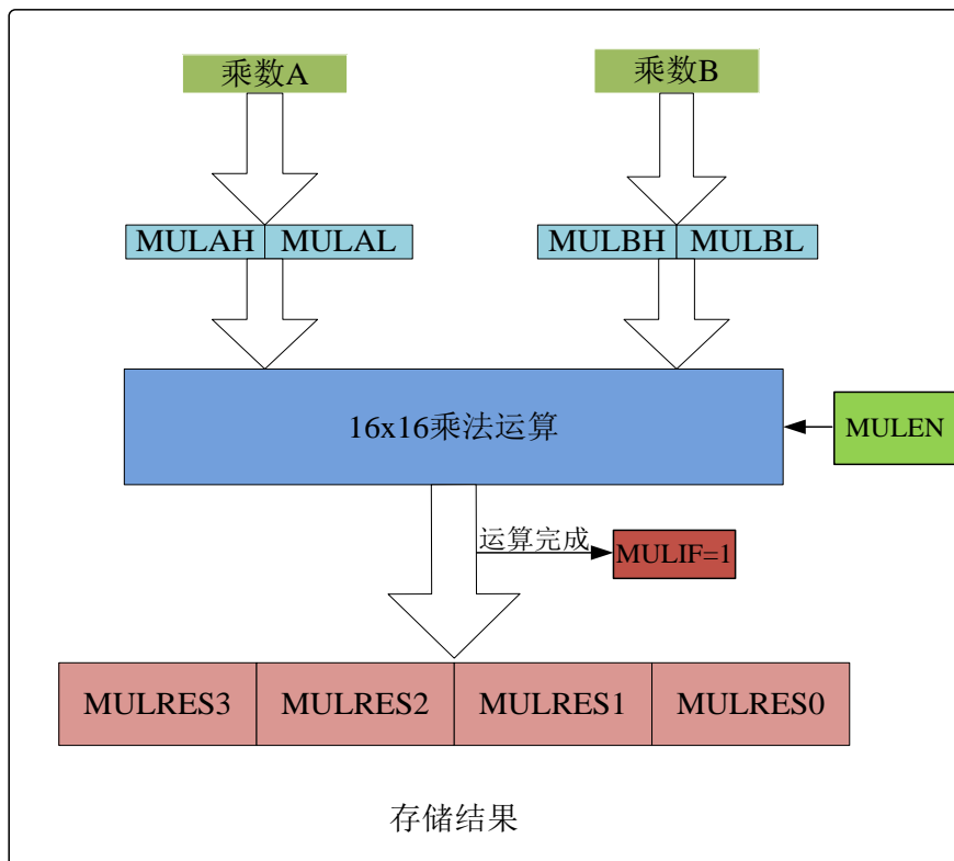
图 14.1 16×16 硬件乘法器原理框图
