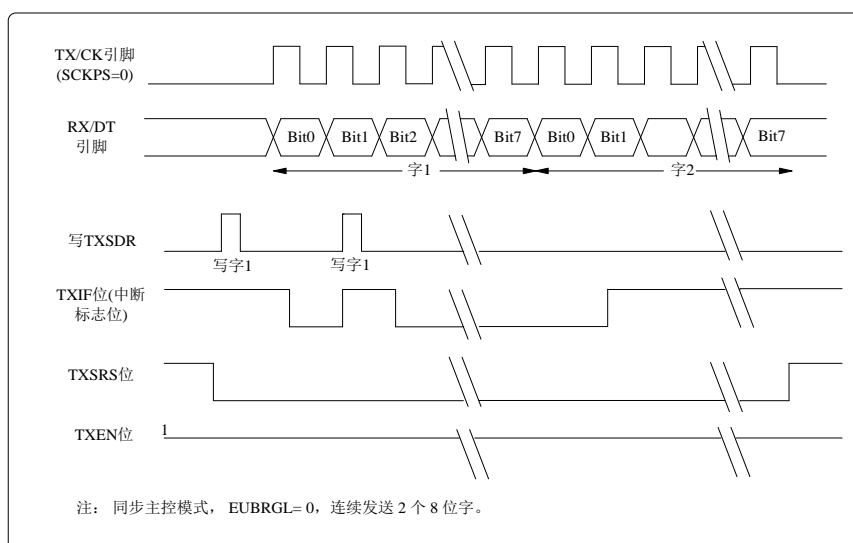
图 11.12 半双工同步发送 (SCKPS x =0)
