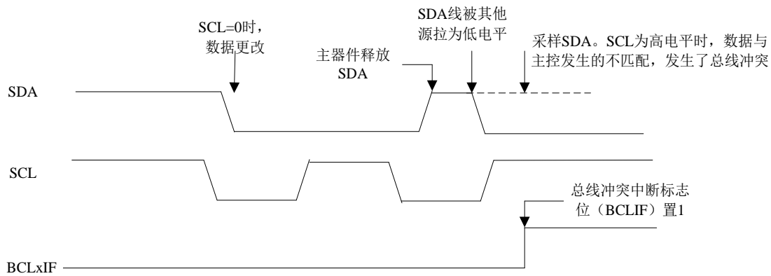
图 10.20 发送和应答时的总线冲突时序
